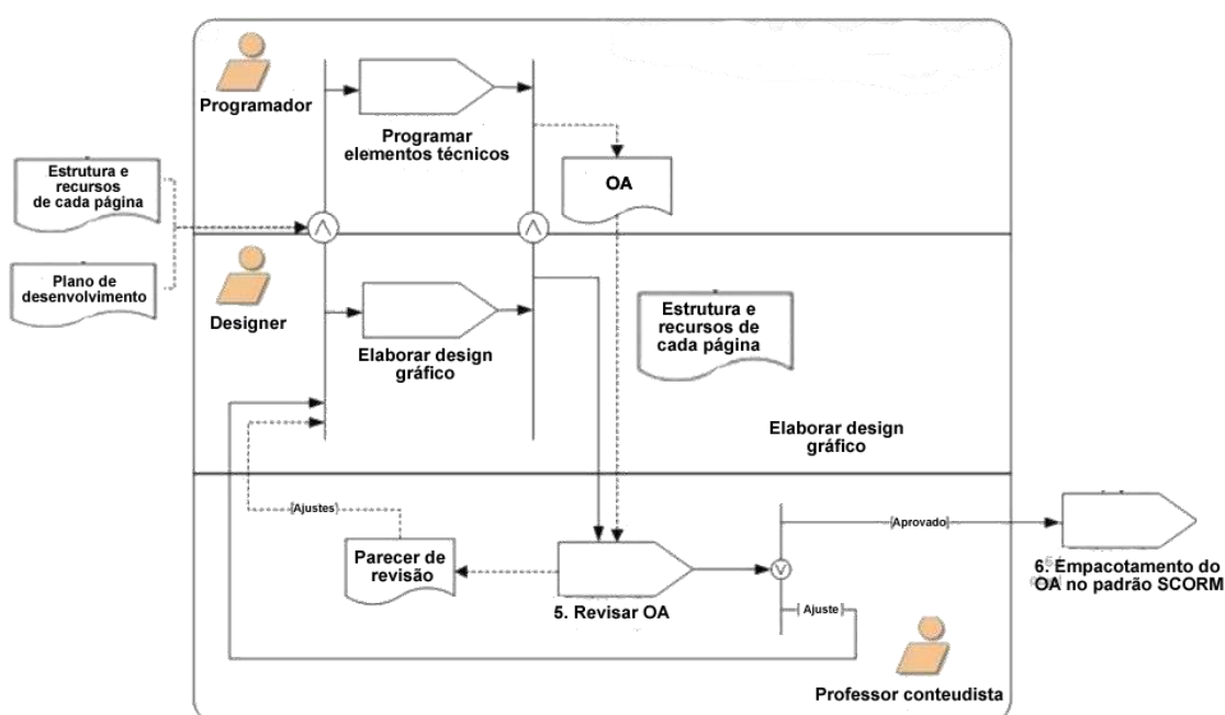
Figura 10 – Processo de Desenvolvimento de um OA Fonte: Pessoa e Benitti (2008, p.6).
