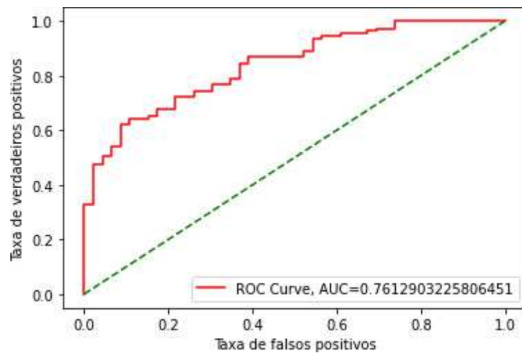
Figura 16 - Curva ROC para o algoritmo de regressão logística
