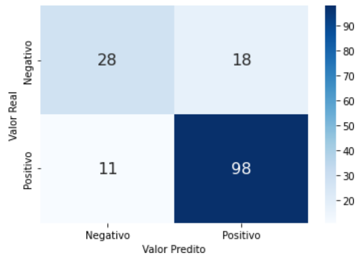
Figura 11 - Matriz de confusão para o algoritmo KNN
