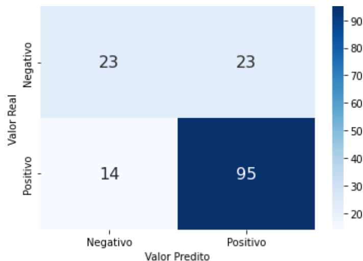
Figura 17 - Matriz de confusão para o algoritmo de regressão logística
