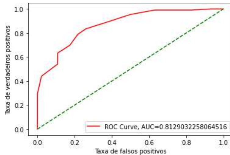
Figura 10 - Curva ROC para o algoritmo KNN
