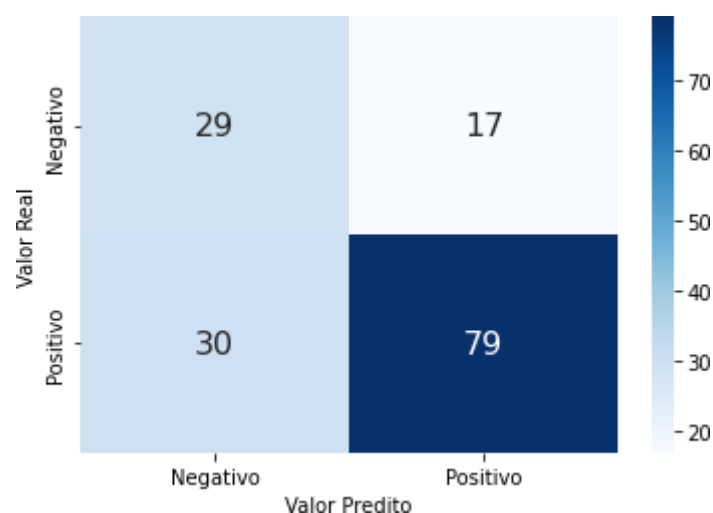
Figura 9 - Matriz de confusão para o algoritmo Naïve Bayes
