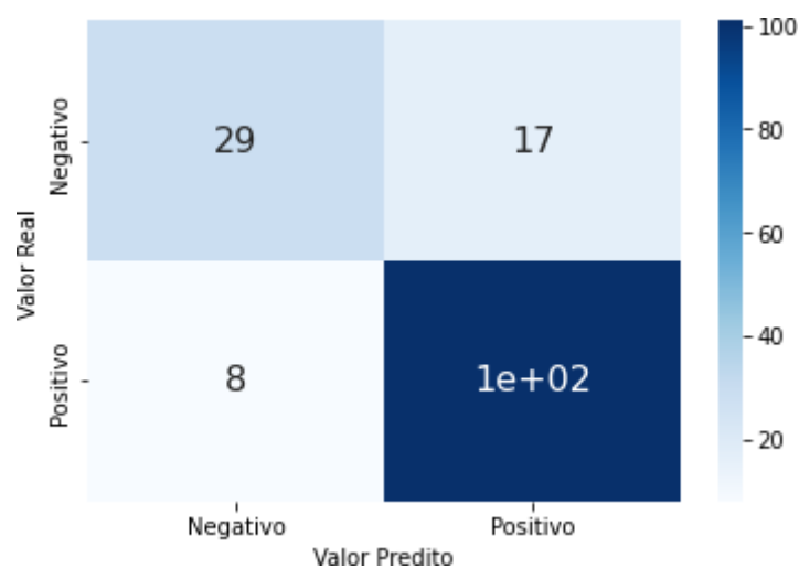
Figura 15 - Matriz de confusão para o algoritmo KSVM
