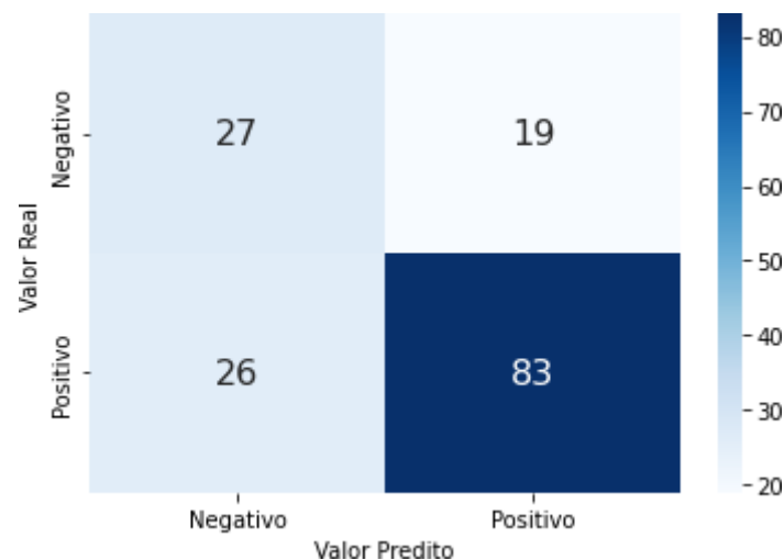
Figura 19 - Matriz de confusão para o algoritmo de árvore de decisão
