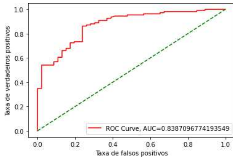
Figura 14 - Curva ROC para o algoritmo KSVM
