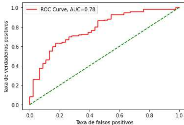
Figura 8 - Curva ROC para o algoritmo Naïve Bayes
