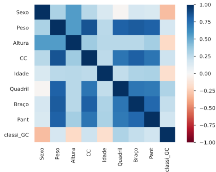
Figura 1 - Correlação de Spearman
