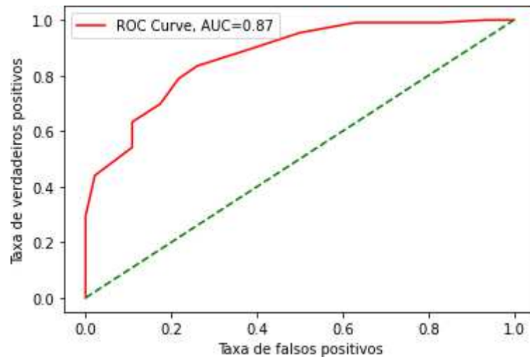
Figura 12 - Curva ROC para o algoritmo L-SVM
