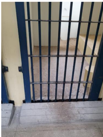
Figura 3 - Base de concreto contra descarrilamento da grade da cela
