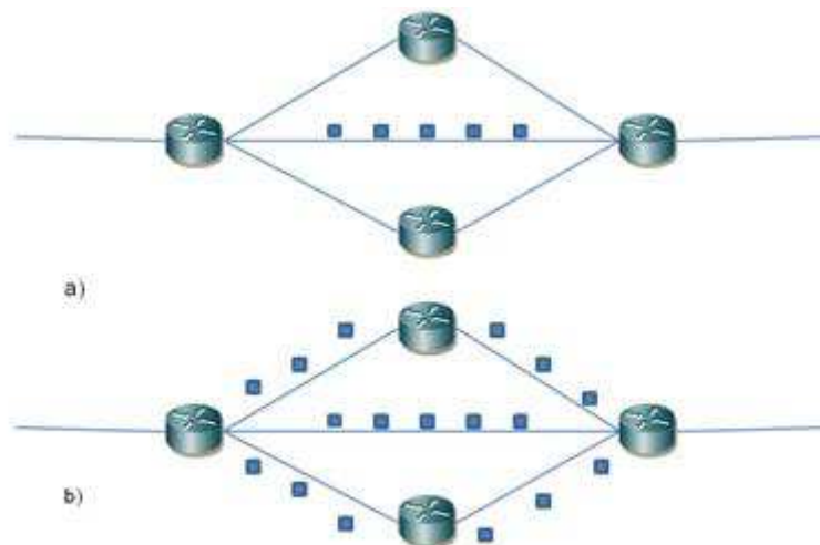
Figura 1: a) Sem engenharia de tráfego; b) Com engenharia de tráfego.
