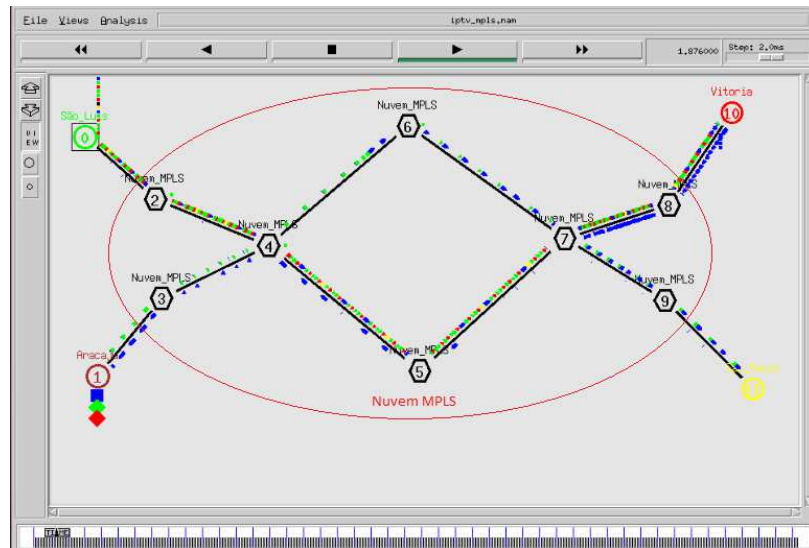
Figura 13: Topologia da empresa implementada na ferramenta.
