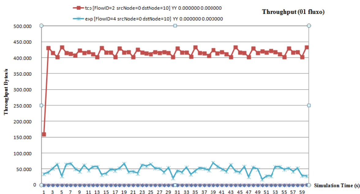
Figura 19: Throughput IPTV x TCP (um fluxo)
