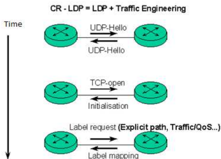
Figura 3: Funcionamento da troca de mensagens do protocolo CR-LDP.
