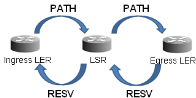
Figura 4: Funcionamento da troca de mensagens do protocolo RSVP-TE.
