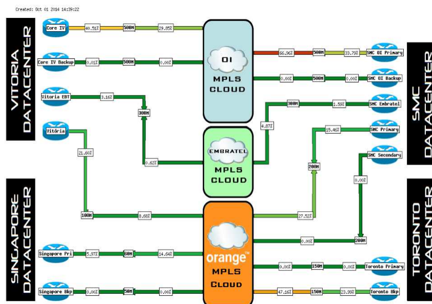
Figura 7: Topologia Corporativa.
