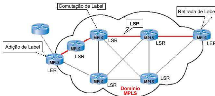
Figura 2: Elementos de uma rede MPLS
