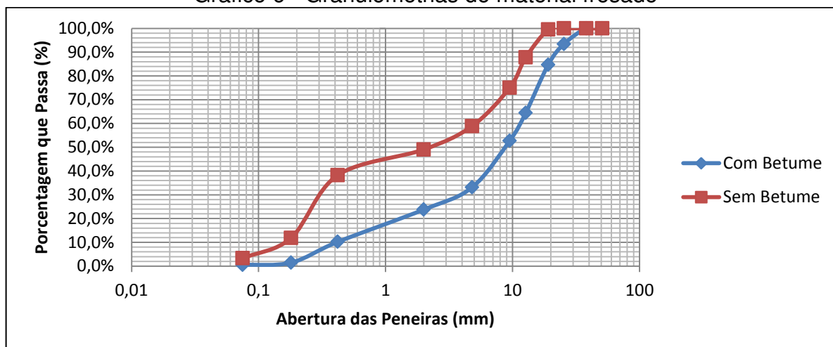
Gráfico 6 - Granulometrias do material fresado
