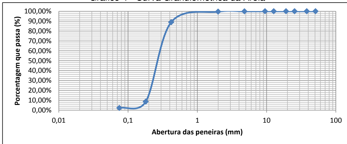
Gráfico 4 - Curva Granulométrica da Areia
