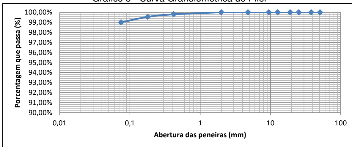
Gráfico 5 - Curva Granulométrica do Fíler
