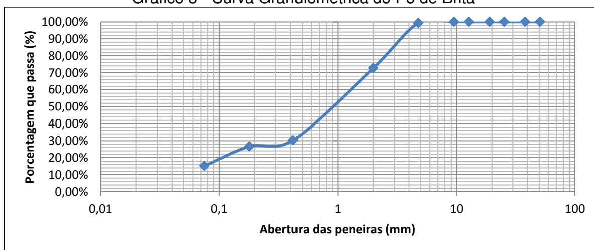
Gráfico 3 - Curva Granulométrica do Pó de Brita
