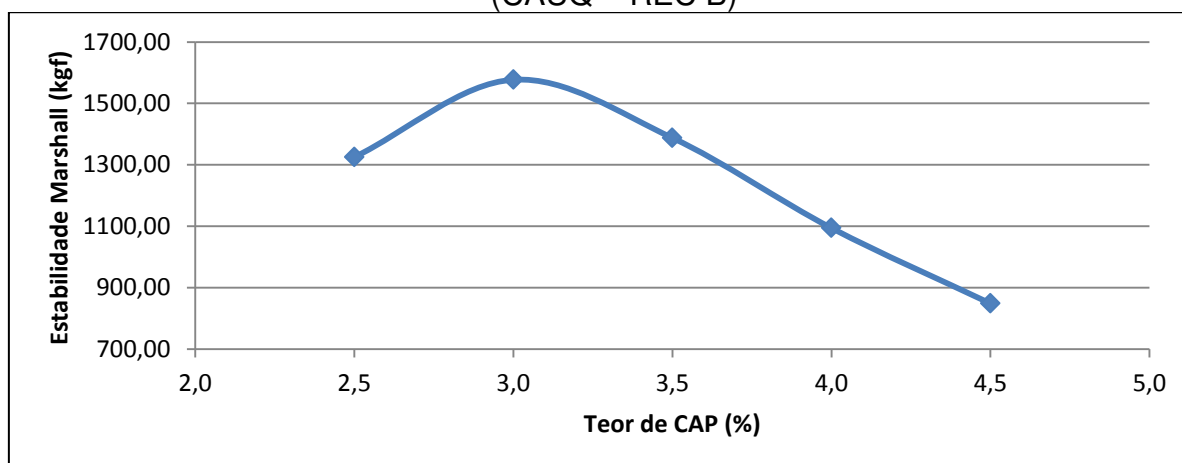
Gráfico 13 - Variação da Estabilidade em Função da Variação do Teor de CAP (CAUQ – REC B)
