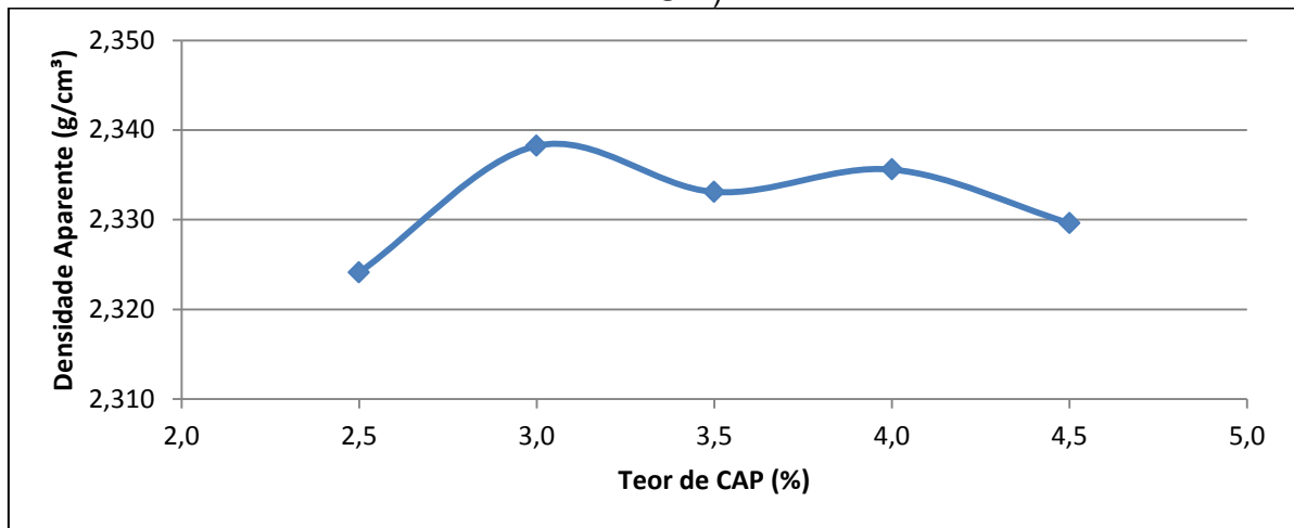
Gráfico 10 - Variação da Dap em Função da Variação do Teor de CAP (CAUQ – REC A)
