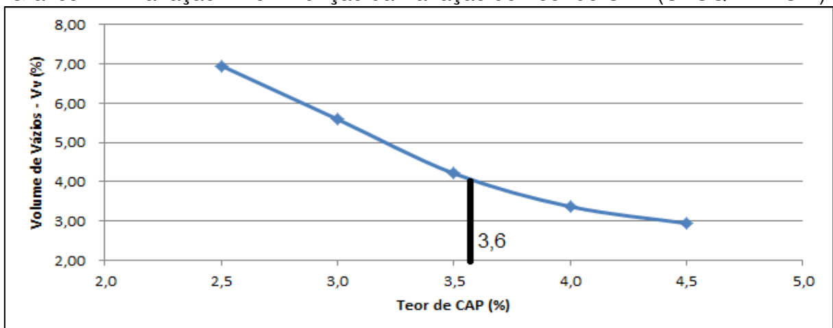
Gráfico 11 - Variação Vv em Função da Variação do Teor de CAP (CAUQ – REC A)
