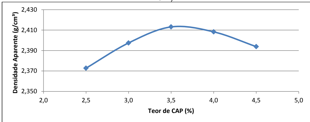
Gráfico 14 - Variação de Dap em Função da Variação do Teor de CAP (CAUQ – REC B)
