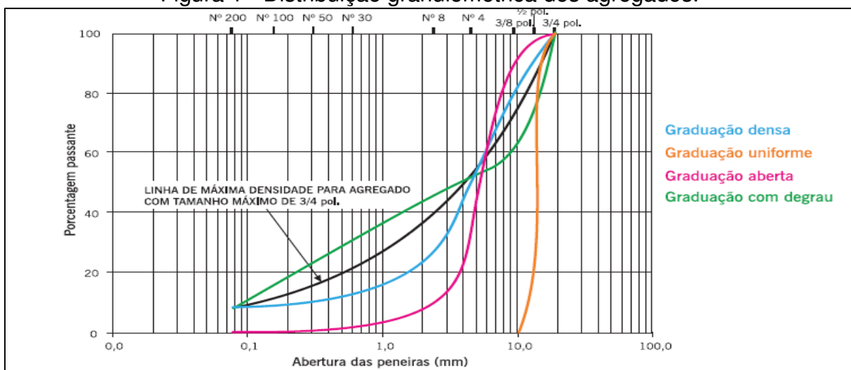
Figura 1 - Distribuição granulométrica dos agregados.
