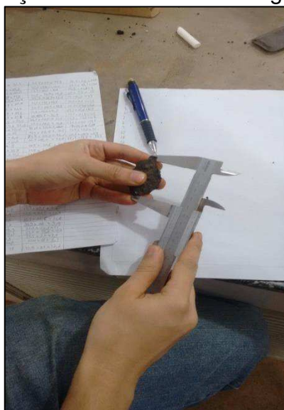
Figura 30 - Medição das Dimensões do Agregado Fresado
