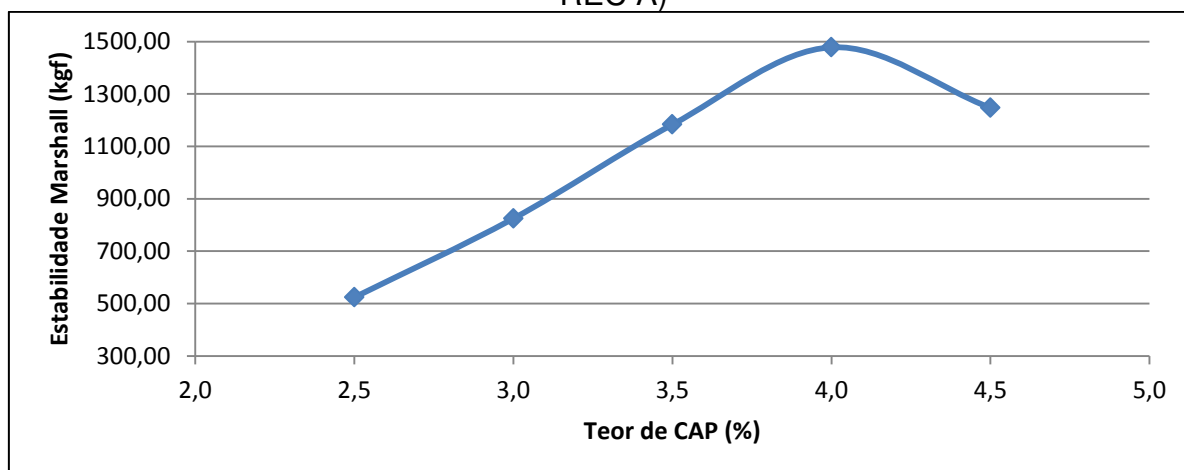
Gráfico 9 - Variação da estabilidade em função da variação do teor de CAP (CAUQ – REC A)
