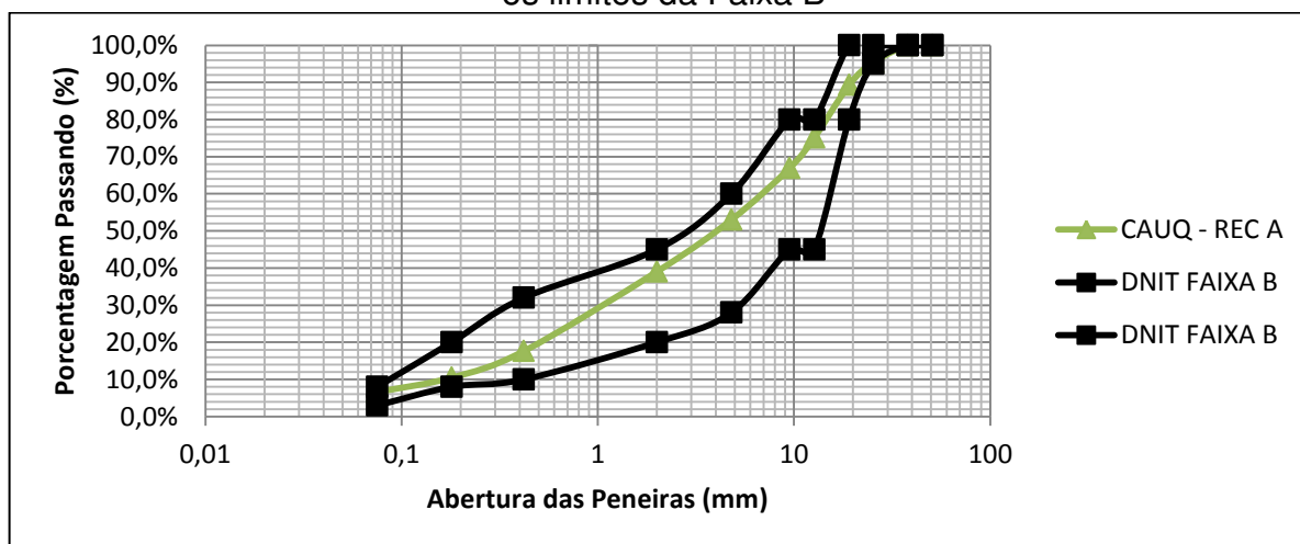
Gráfico 7 - Comparação entre a curva granulométrica da mistura CAUQ – REC A e os limites da Faixa B
