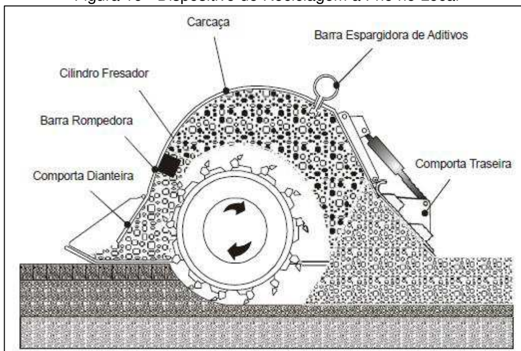
Figura 16 - Dispositivo de Reciclagem a Frio no Local
