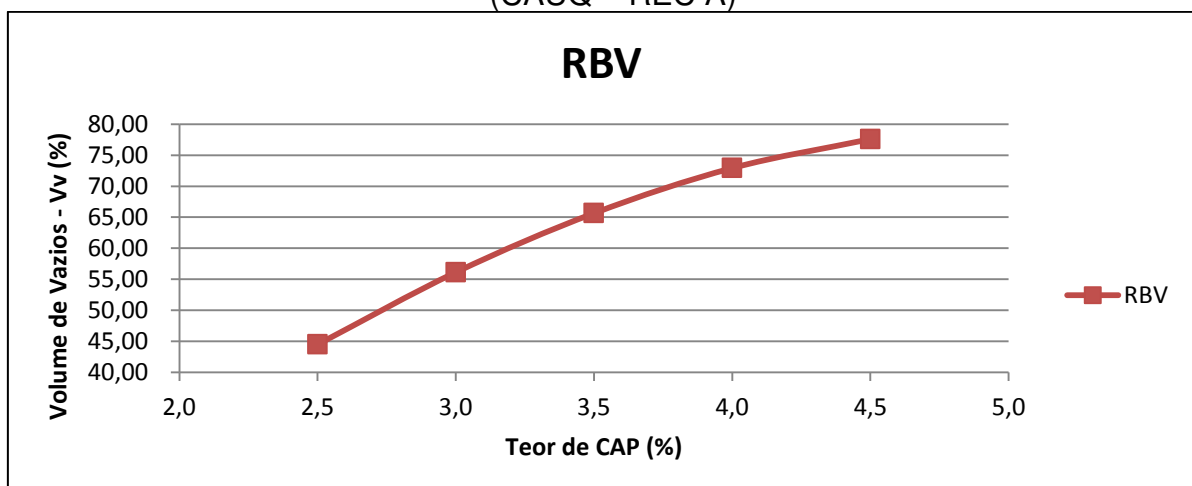
Gráfico 12 - Variação de Vv e de RBV em Função da Variação do Teor de CAP (CAUQ – REC A)
