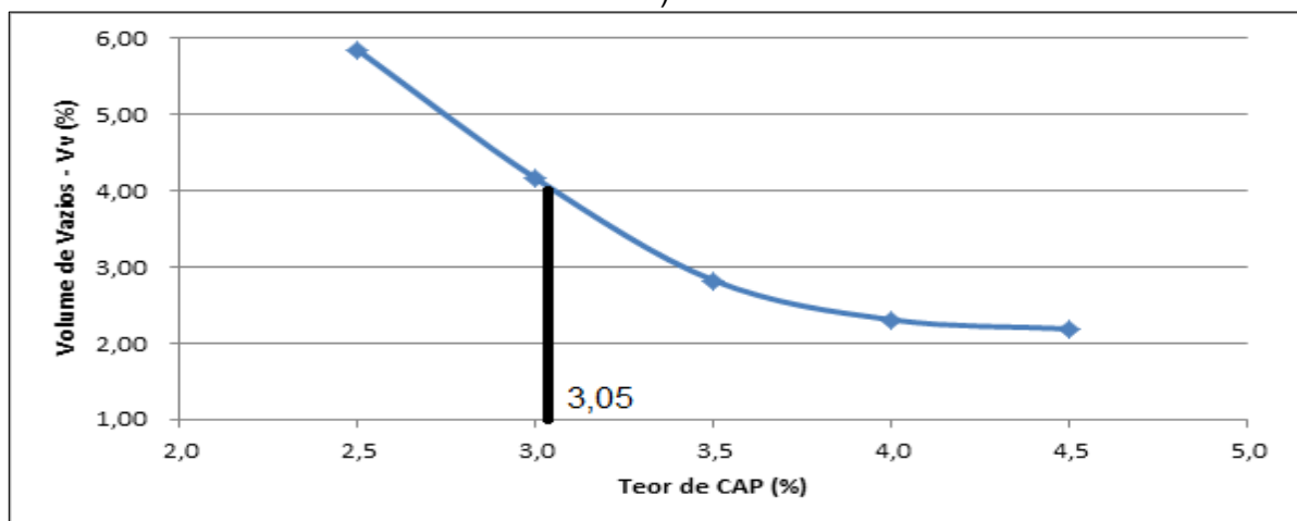
Gráfico 15 - Variação de Vv em Função da Variação do Teor de CAP (CAUQ – REC B)
