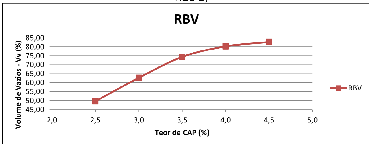
Gráfico 16 - Variação de Vv e RBV em Função da Variação do Teor de CAP (CAUQ – REC B)
