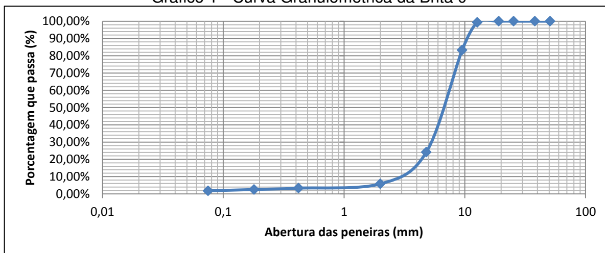
Gráfico 1 - Curva Granulométrica da Brita 0
