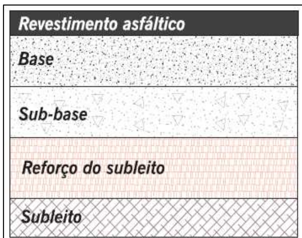
Figura 4 - Estrutura de Pavimento Flexível Figura 5 - Rodovia de Pavimento Flexível
