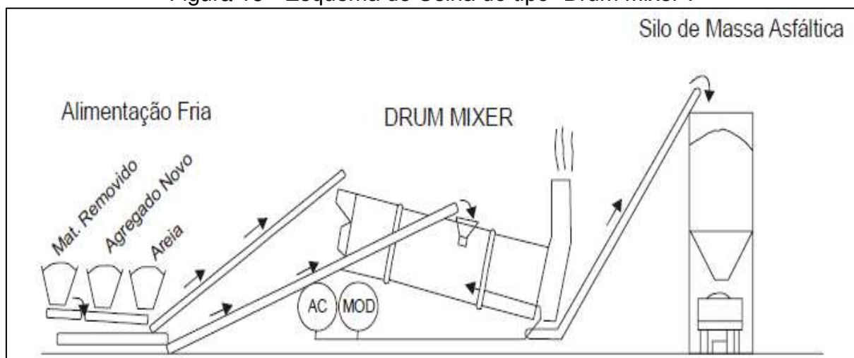
Figura 15 - Esquema de Usina do tipo “Drum Mixer”.
