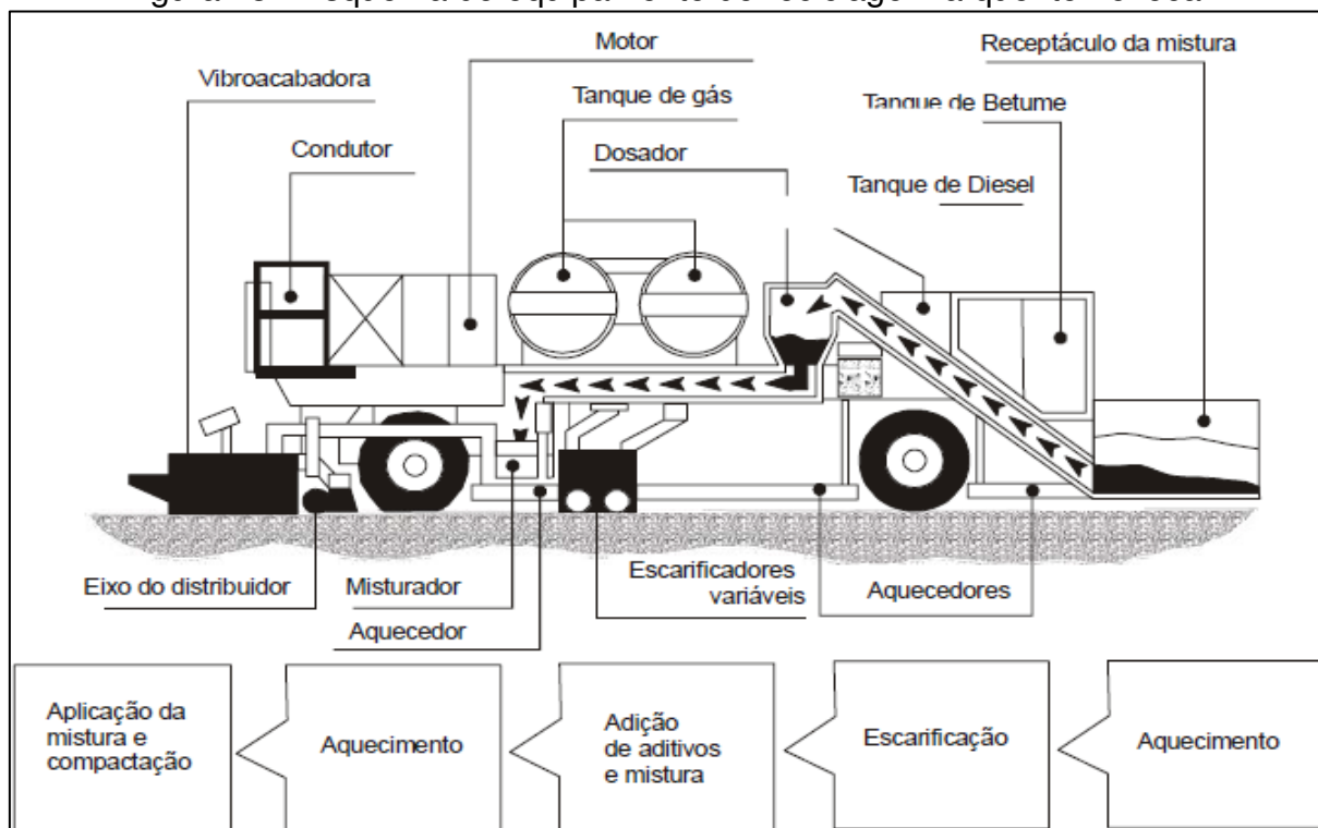
Figura 13 - Esquema do equipamento de reciclagem a quente no local
