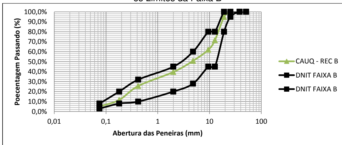
Gráfico 8 - Comparação Entre a curva granulométrica da mistura CAUQ –REC B e os Limites da Faixa B
