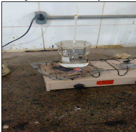
Figura 19 - Realização do ensaio do ponto de amolecimento
