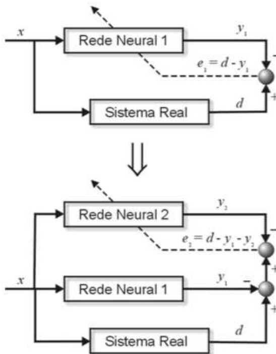
Figura 2.14: Arranjo de MRNA com duas redes
