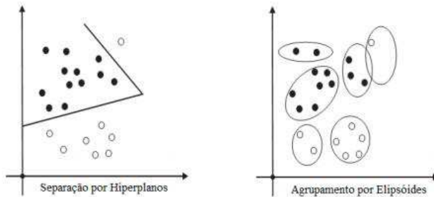
Figura 2.10: Classificação com redes MLP(esquerda) e redes RBF(direita)
