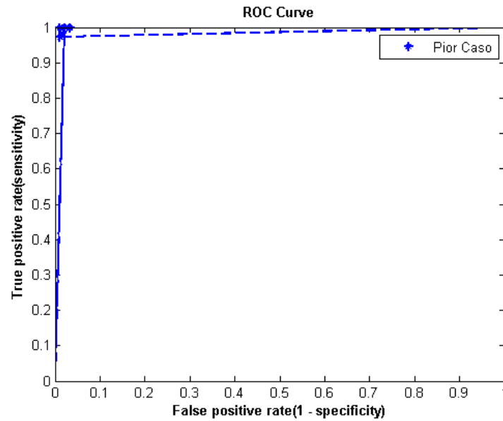
Figura 3.3: Curva ROC (Pior Caso)– Base de dados 1
