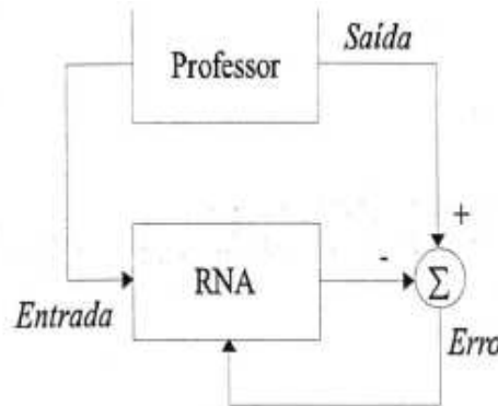
Figura 2.7: Aprendizado supervisionado
