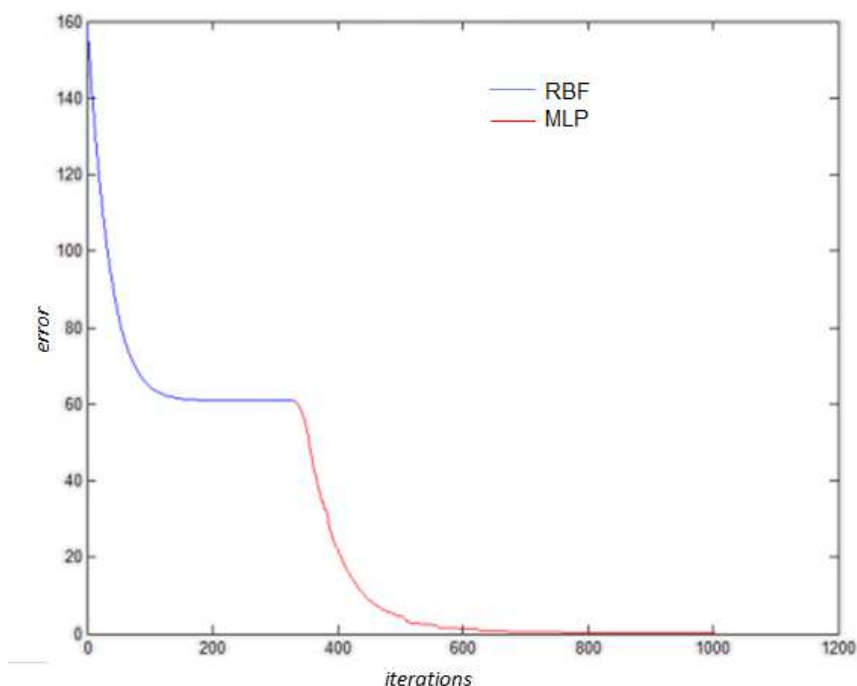
Figura 3.1: Gráfico do Erro Quadrático Médio
