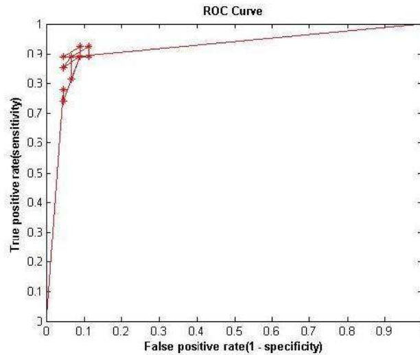
Figura 6. Curva ROC – Base de Dados 2
