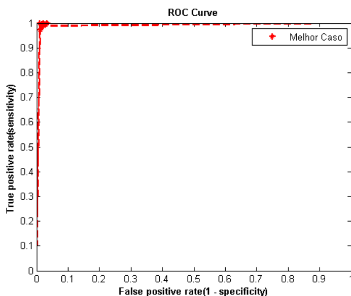
Figura 3.2: Curva ROC (Melhor Caso) – Base de dados 1
