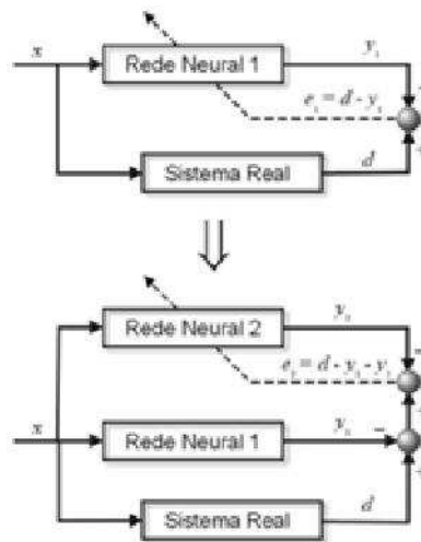
Figura 3. Arranjo de MRNA com duas redes.
