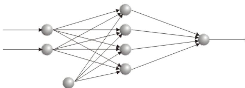
Figura 2.6: RNA com uso de bias
