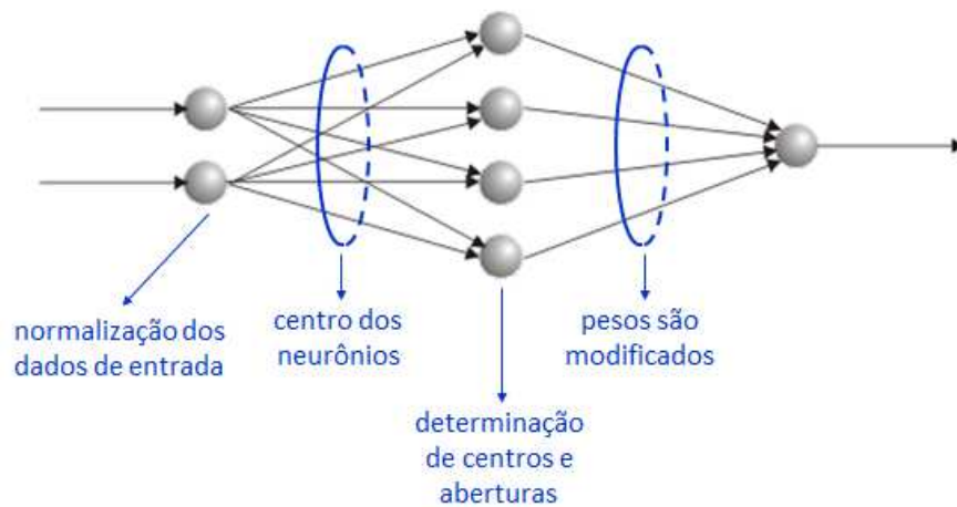
Figura 2.9: Estrutura da RNA do tipo RBF
