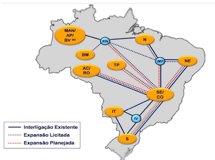
FIGURA 1: Representação esquemática para as interligações entre os 3 subsistemas nacionais (SIN).
