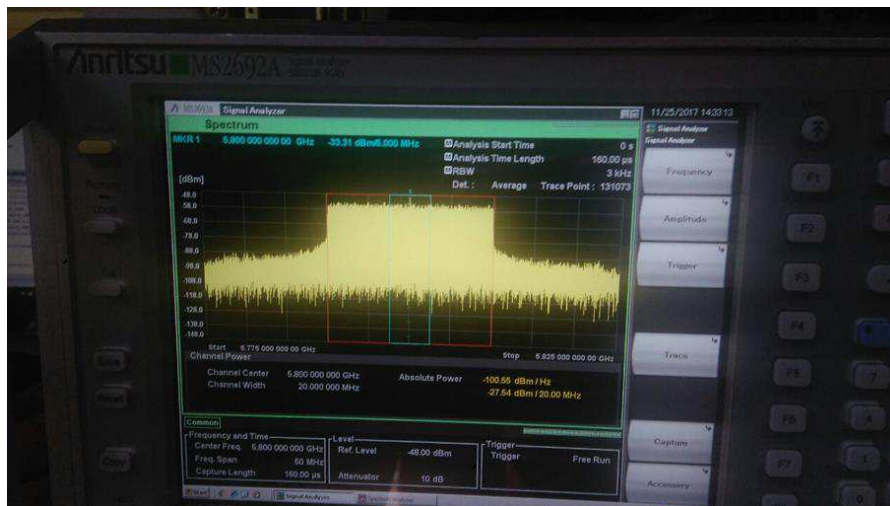
Figura 53: Sinal OFDM capturado durante as campanhas de medições.
