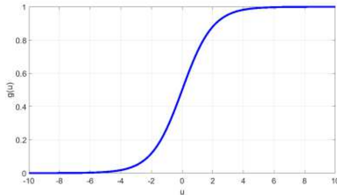
Figura 23: Função logística.
