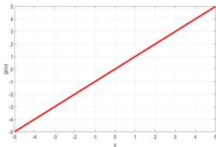
Figura 26: Função linear.
