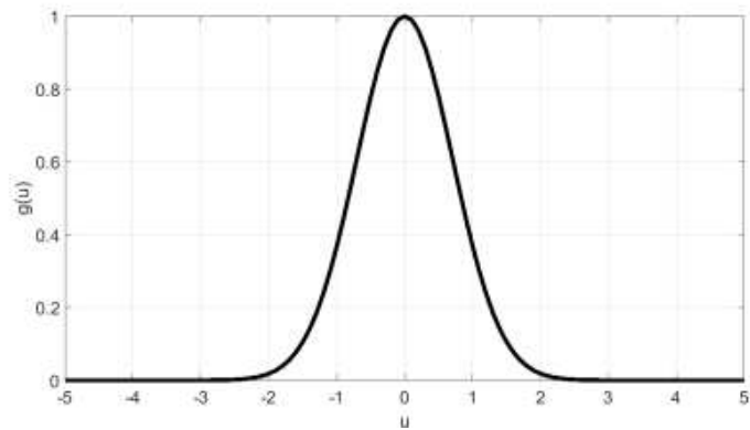
Figura 25: Função Gaussiana.
