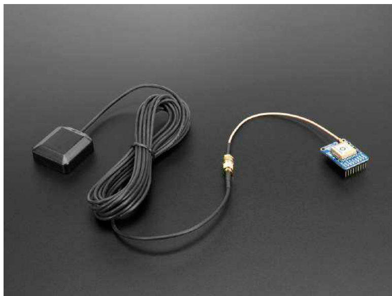
FIGURA 5.20 – Receptor ligado a uma antena GPS automotiva.
