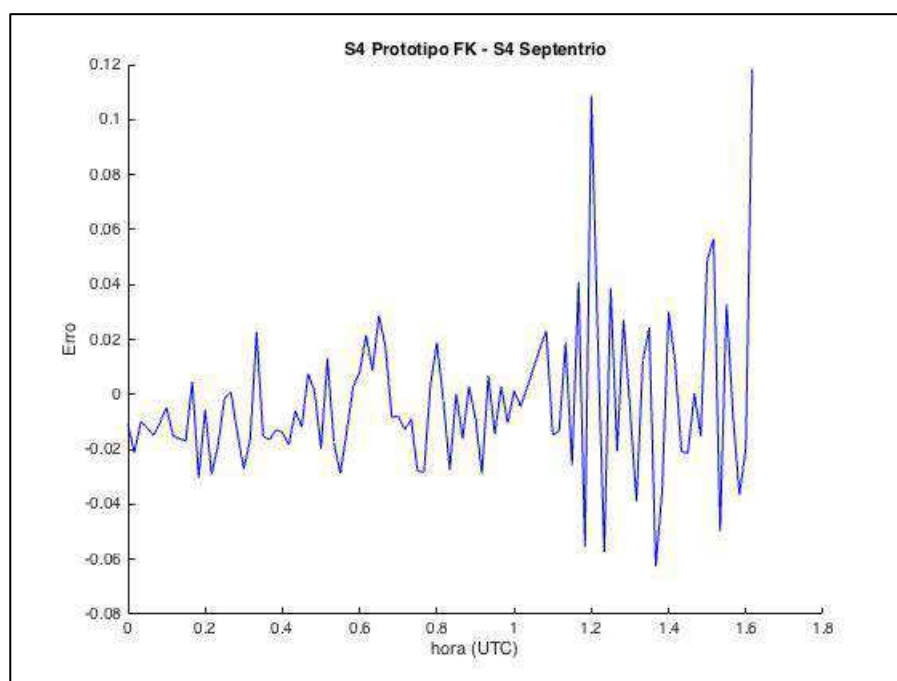
FIGURA 6.7 – Erro na estimativa do índice S_{4FK}^* pelo protótipo em relação ao monitor profissional após uso do Filtro de Kalman.
