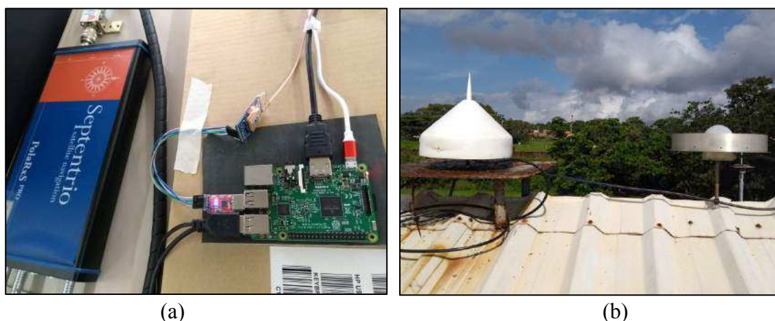
FIGURA 5.3 – a) Protótipo do monitor de cintilação ionosférica ao lado do Septentrio. b) Antenas GNSS helicoidais Choke-ring instaladas sobre o prédio do INPE. À esquerda, a antena do monitor Septentrio e à direita, a antena do protótipo.
