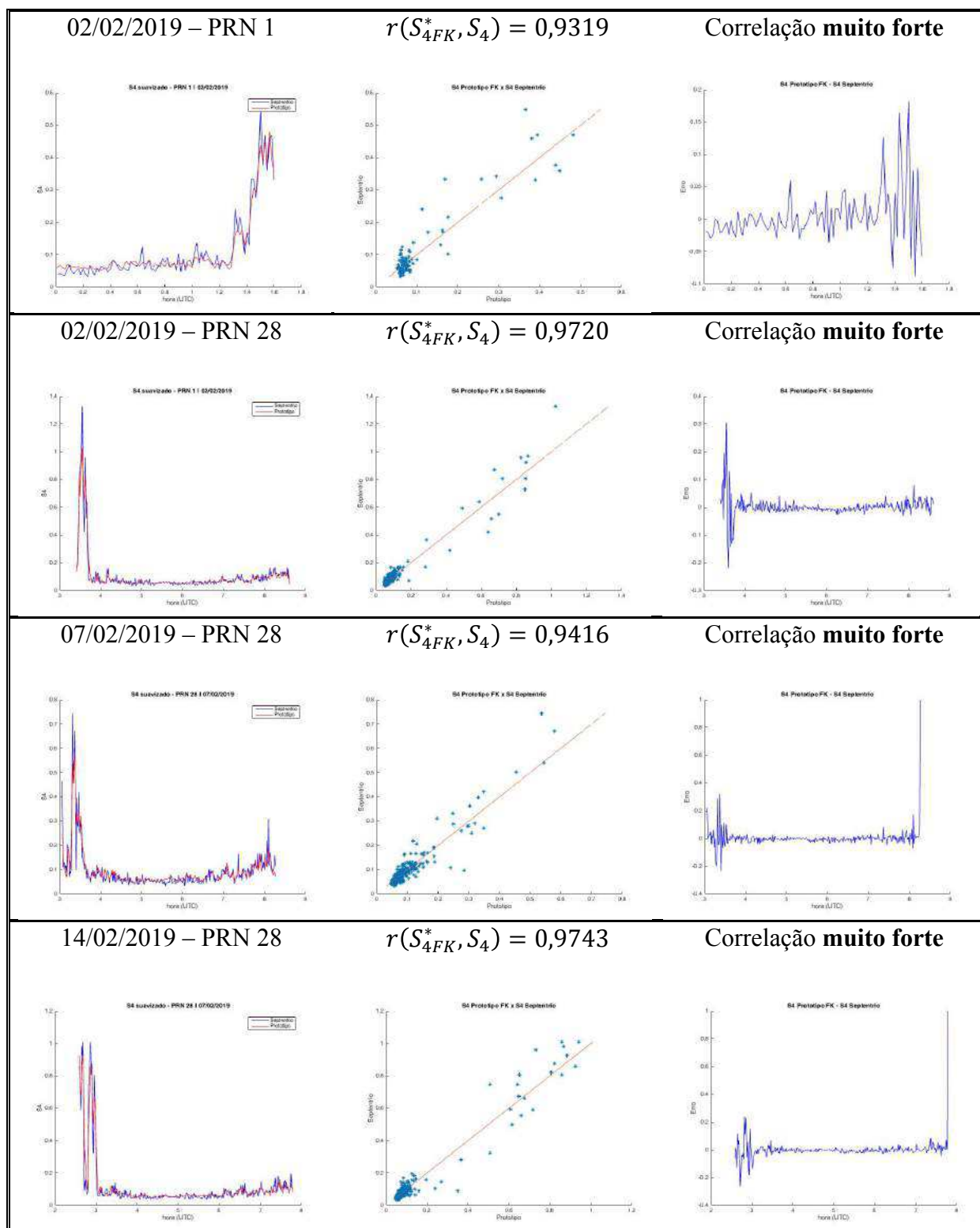
FIGURA 6.9 – Comparação entre os índices S4 obtidos pelo protótipo e pelo monitor profissional após aplicação do filtro de Kalman.
