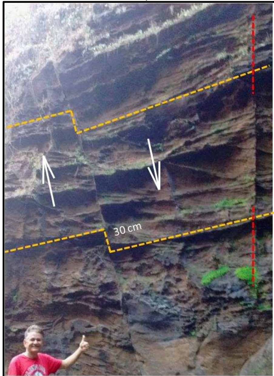
FIGURA 50: Falha de cisalhamento em tesoura com deslocamento vertical localizada no interior do paredão de arenito dentro do canion da cachoeira do Macapá.
