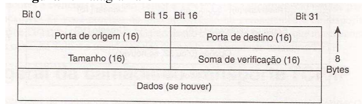
Figura 2: Datagrama UDP
