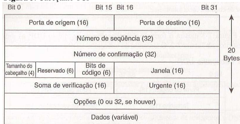
Figura 3: Cabeçalho TCP
