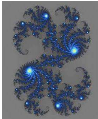
Figura 20: Representação do Conjunto de Julia para um determinado valor de c .
