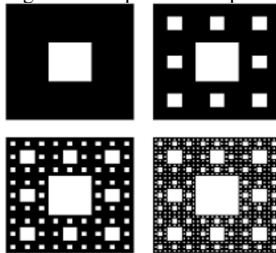
Figura 16: Tapete de Sierpinski
