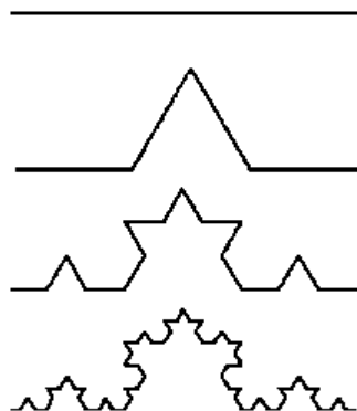
Figura 13: Curva de Koch e uma aplicação
