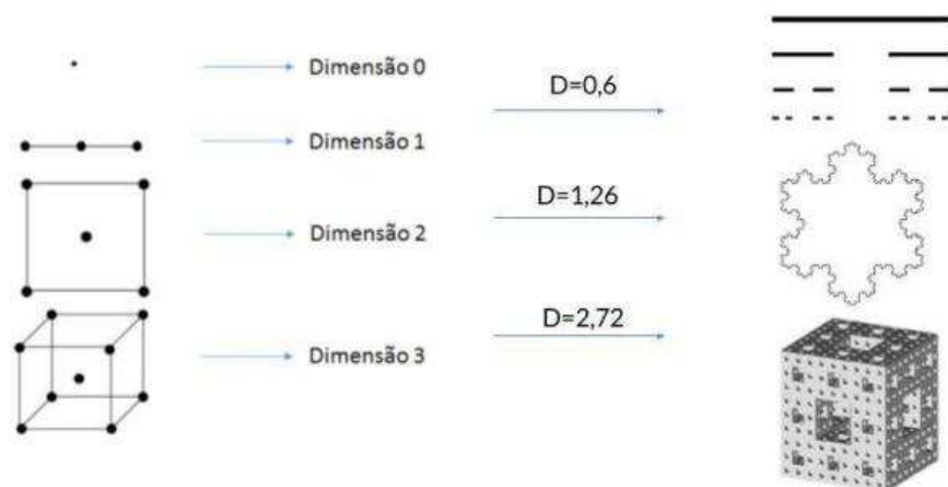
Figura 7: Dimensão euclidiana e dimensão Fractal.
