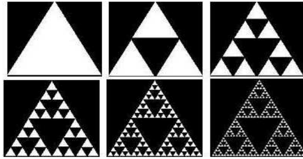
Figura 15: Triângulo de Sierpinski)
