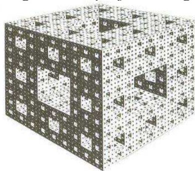
Figura 18: Esponja de Menger
