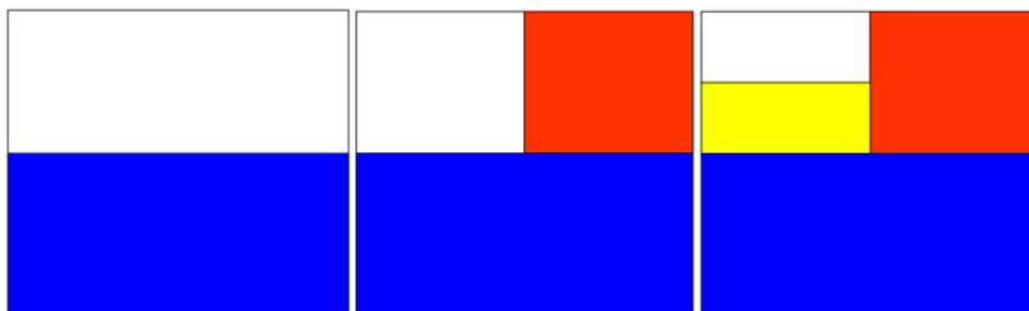
Figura 29: Ideia intuitiva de limites
