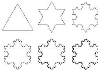
Figura 2: Floco de neve de Koch
