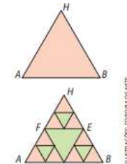
Figura 24: Geometria e Trigonometria: definição de fractal
