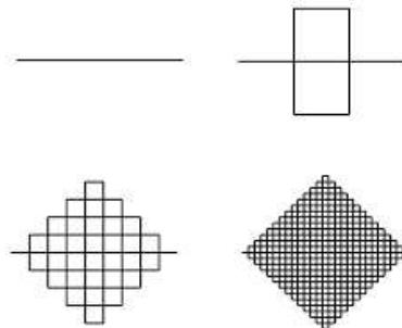
Figura 11: Curva de Peano
