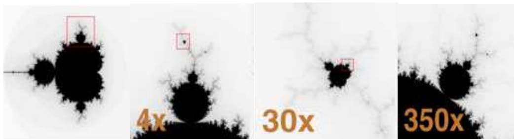
Figura 1: Ampliação 350 vezes do Conjunto de Mandelbrot.
