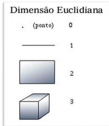
Figura 5: Dimensão Euclidiana.
