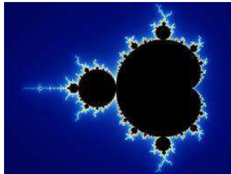
Figura 3: Conjunto de Mandelbrot
