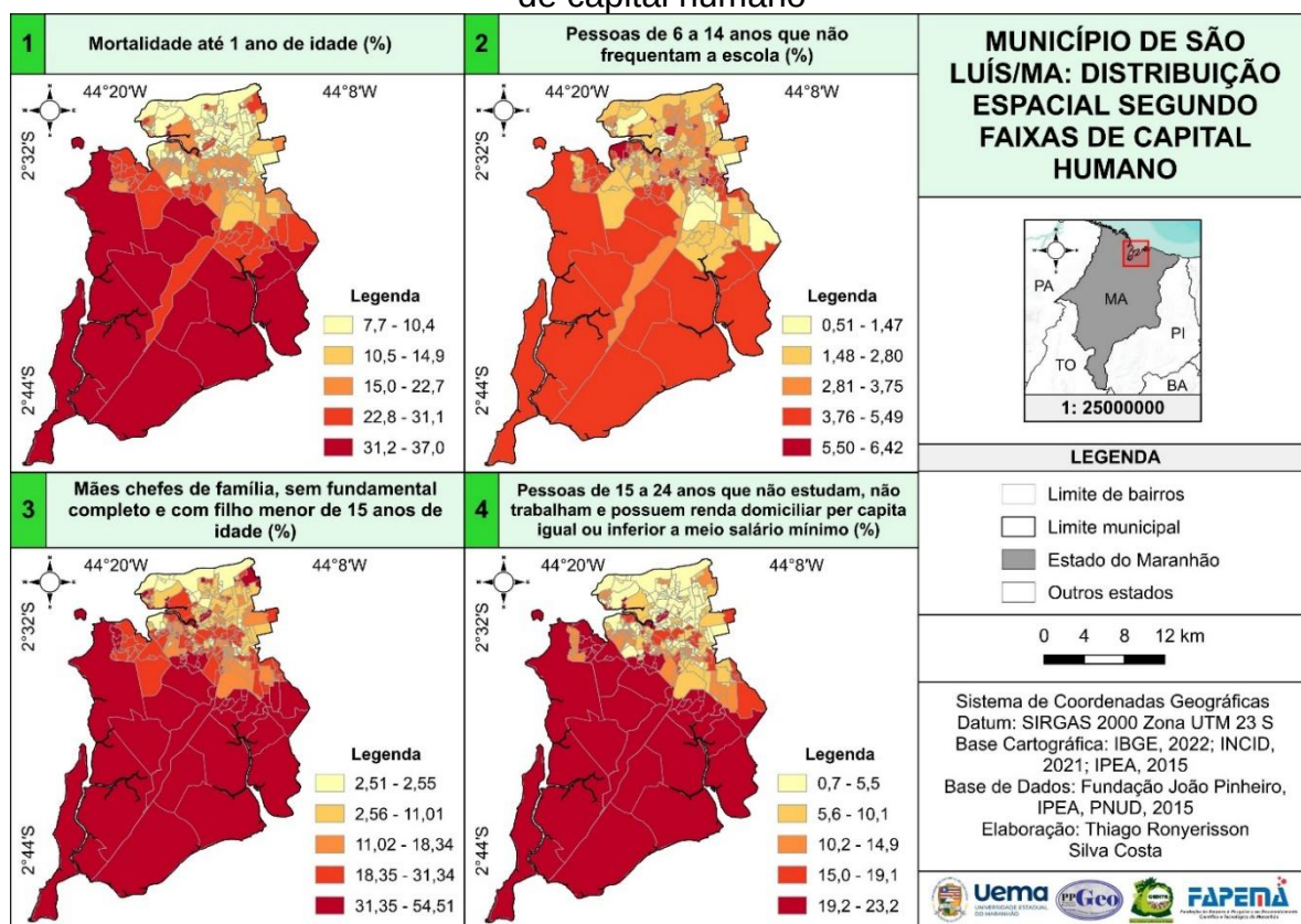
Figura 21 – Município de São Luís, Maranhão: distribuição espacial segundo faixas de capital humano
