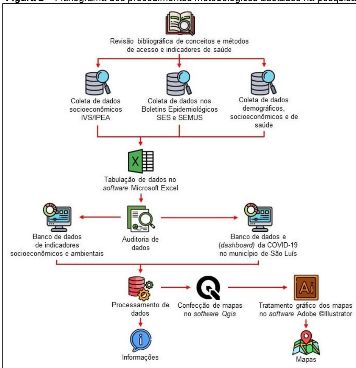
Figura 2 – Fluxograma dos procedimentos metodológicos adotados na pesquisa
