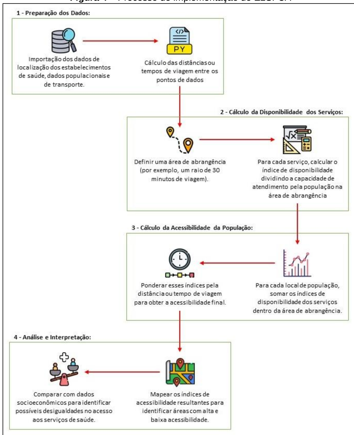
Figura 4 – Processo de implementação do E2SFCA
