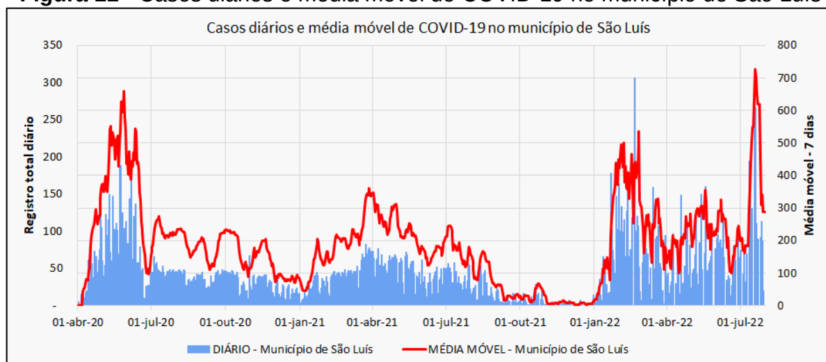
Figura 11 - Casos diários e média móvel de COVID-19 no município de São Luís
