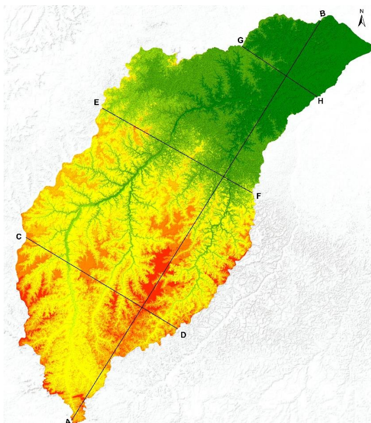
Figura 48 – Identificação e localização dos Perfis Topográficos.
