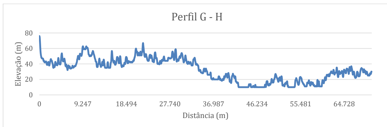
Figura 52 – Perfil topográfico G-H.
