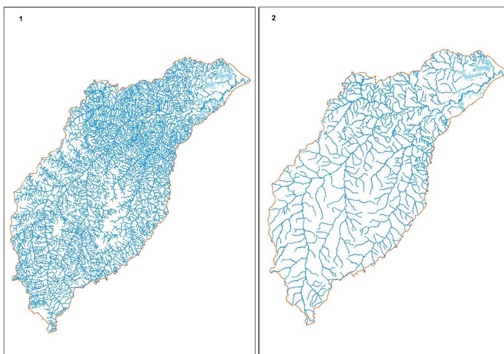
Figura 7 – Diferentes tipos de drenagem utilizadas no trabalho.
