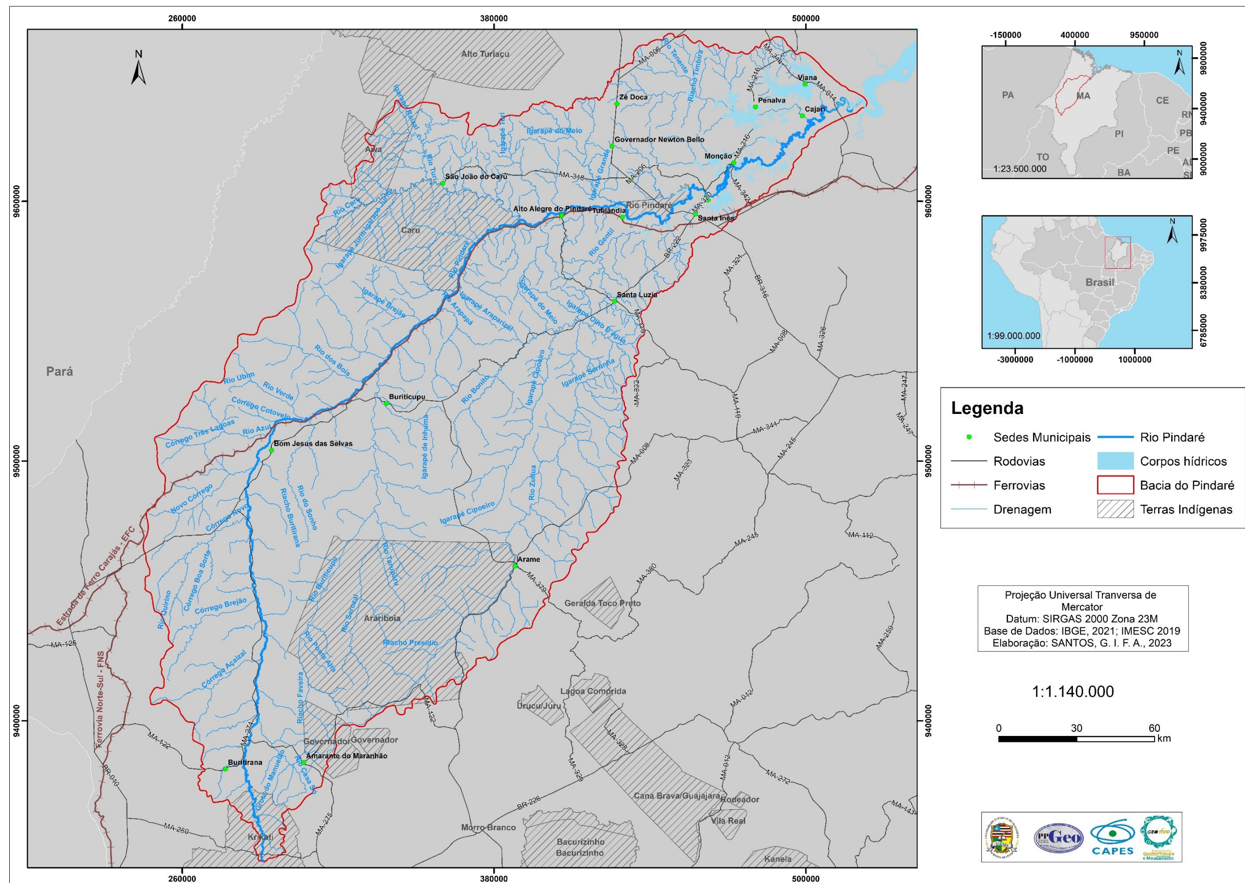
Figura 1 – Localização da Bacia do rio Pindaré – MA.
