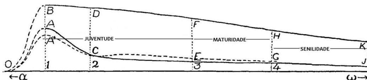
Figura 2 – Fases de desenvolvimento da paisagem.
