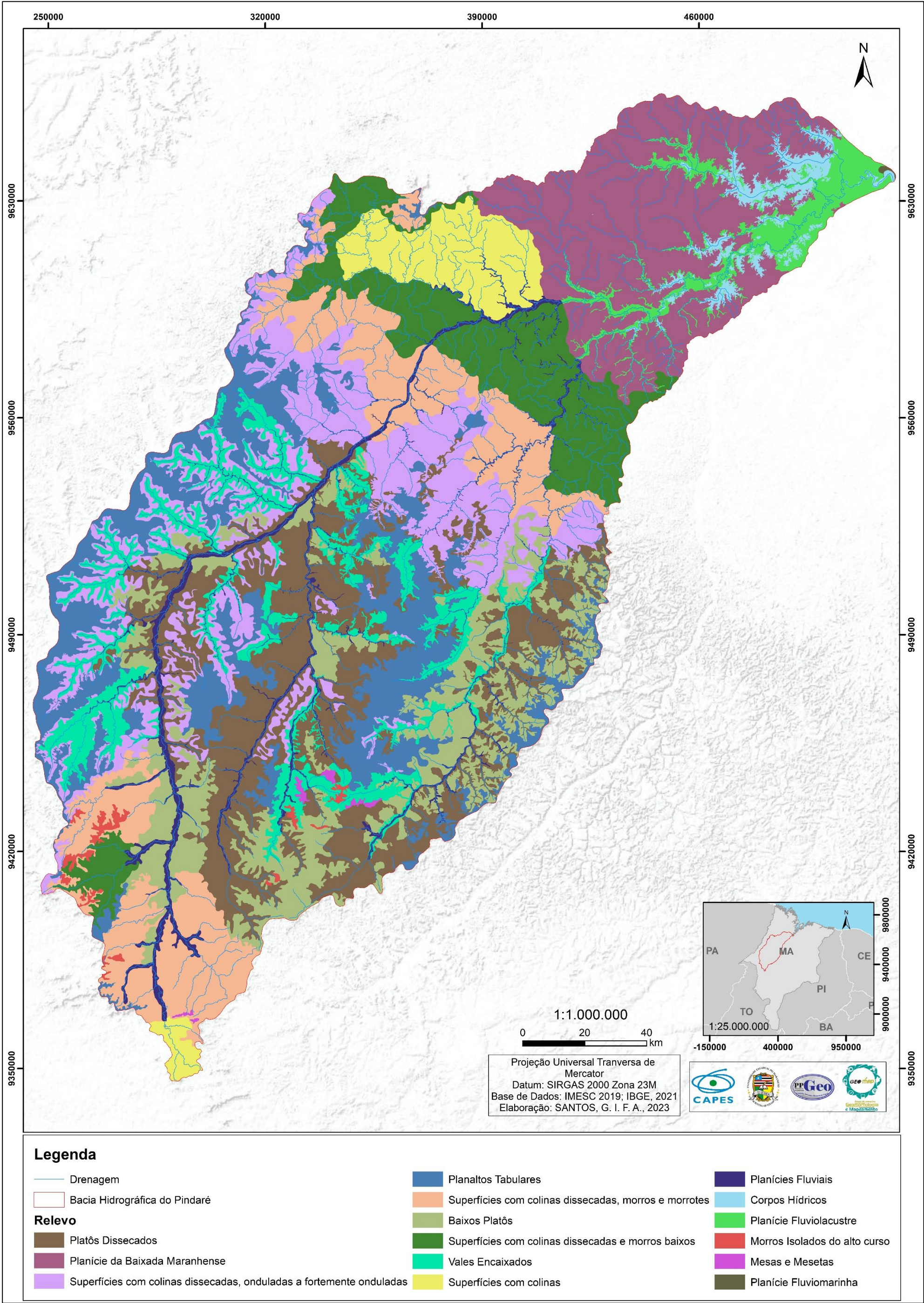
Figura 20—Compartimentos Geomorfológicos da bacia hidrográfica do Pindaré.
