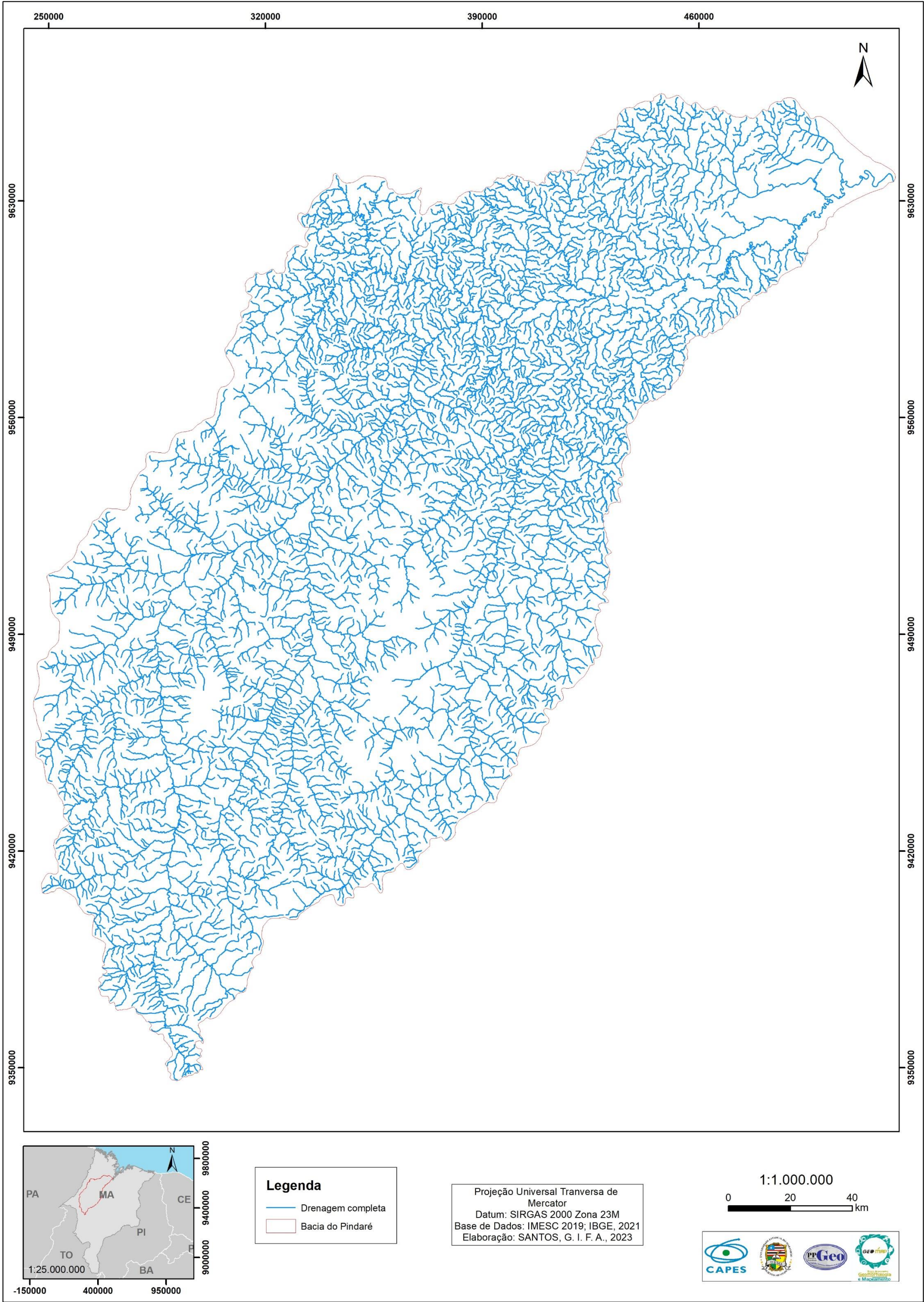
Figura 46 – Drenagem altamente complexa da bacia do rio Pindaré.
