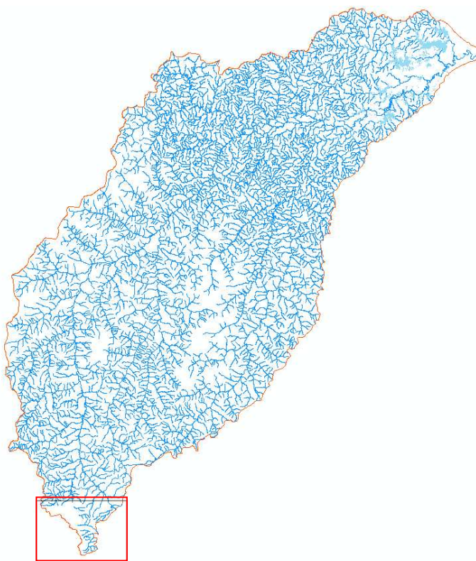
Figura 6 – Preenchimento da lacuna da drenagem no extremo sul da bacia do rio Pindaré, utilizando a rede de drenagem do IBGE (1989), destacado em vermelho.
