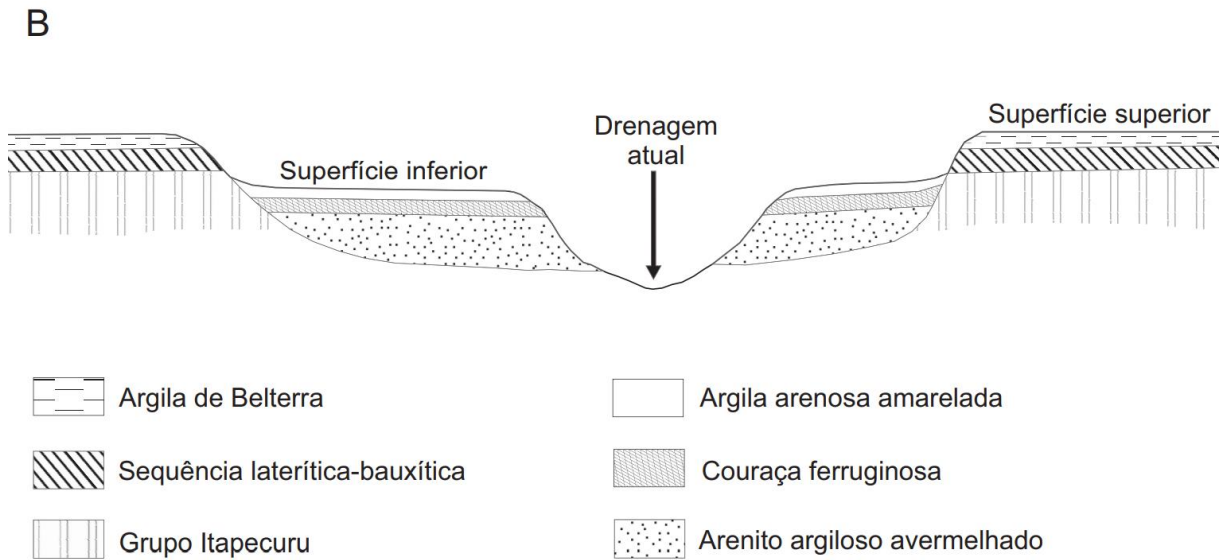
Figura 17 – Representação das superfícies superior e inferior associadas à laterita maduras do Paleógeno e do Neógeno.
