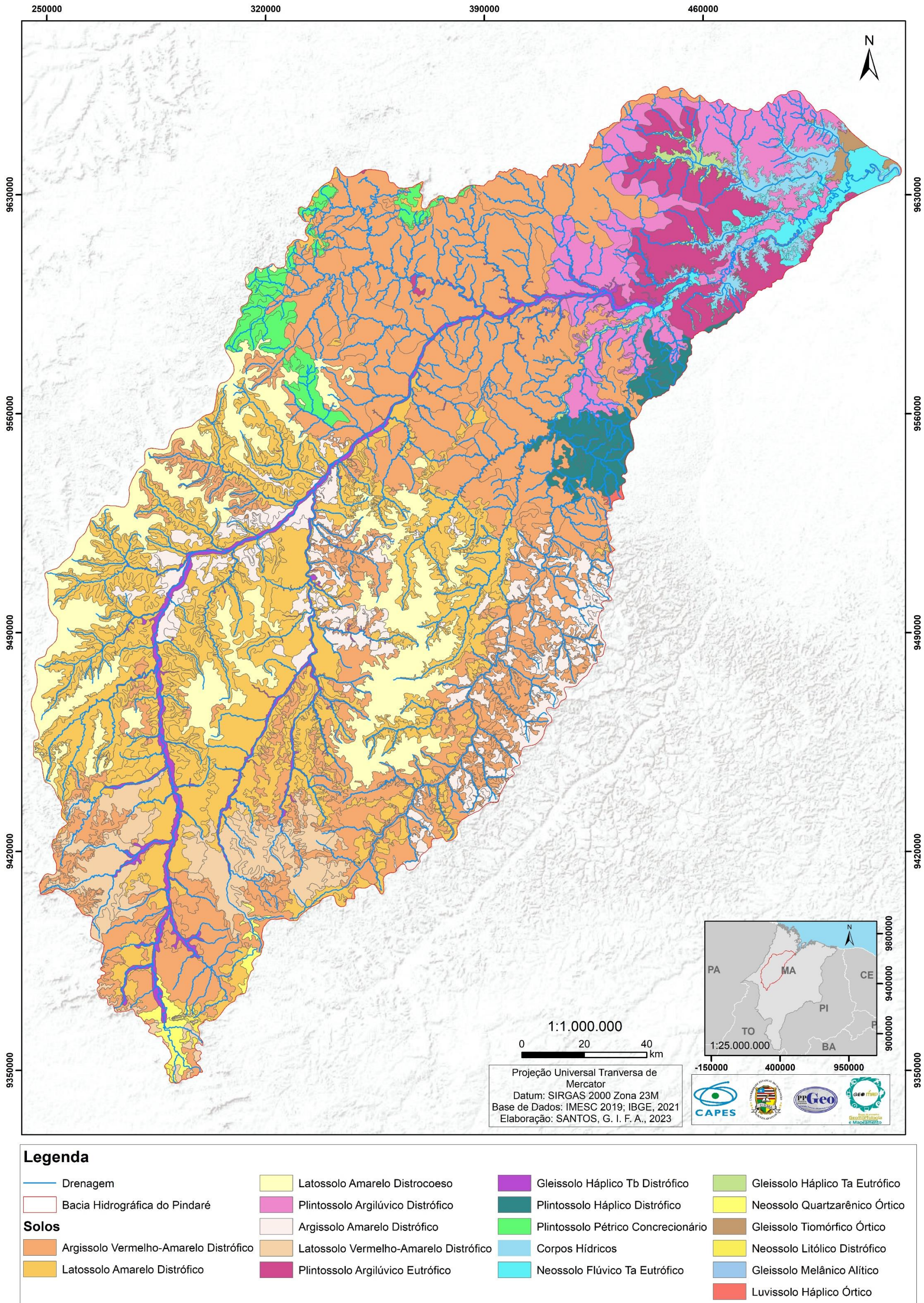
Figura 28 – Mapa de Solos da bacia do rio Pindaré.
