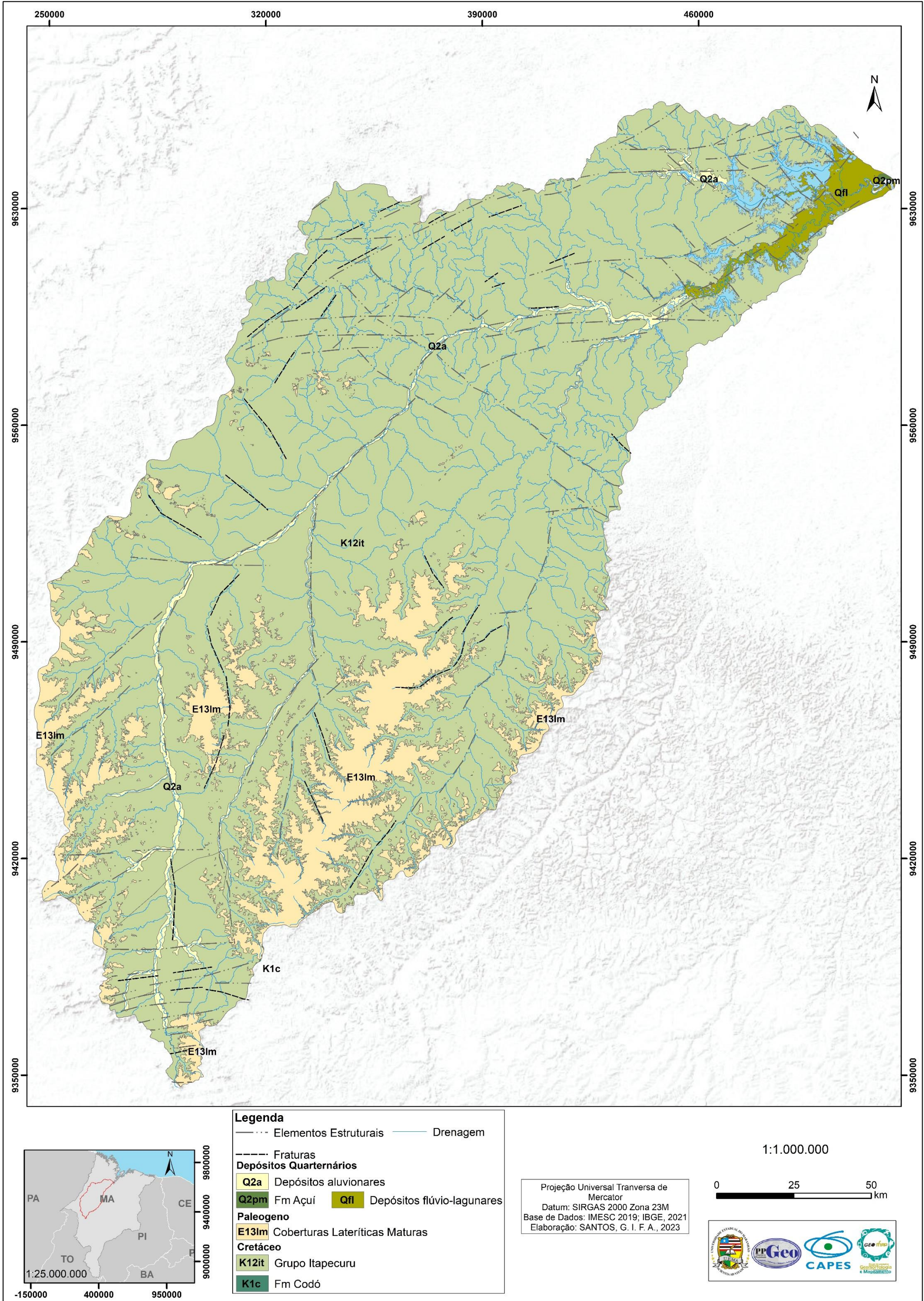
Figura 15– Unidades litoestratigráficas presentes na bacia hidrográfica do rio Pindaré.
