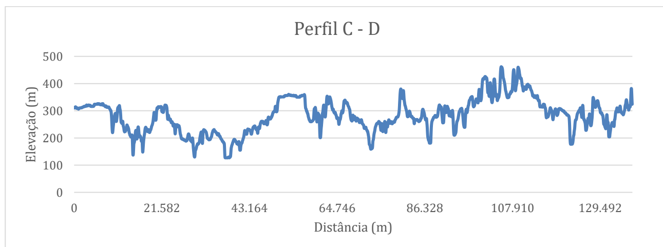
Figura 50 – Perfil topográfico C-D.
