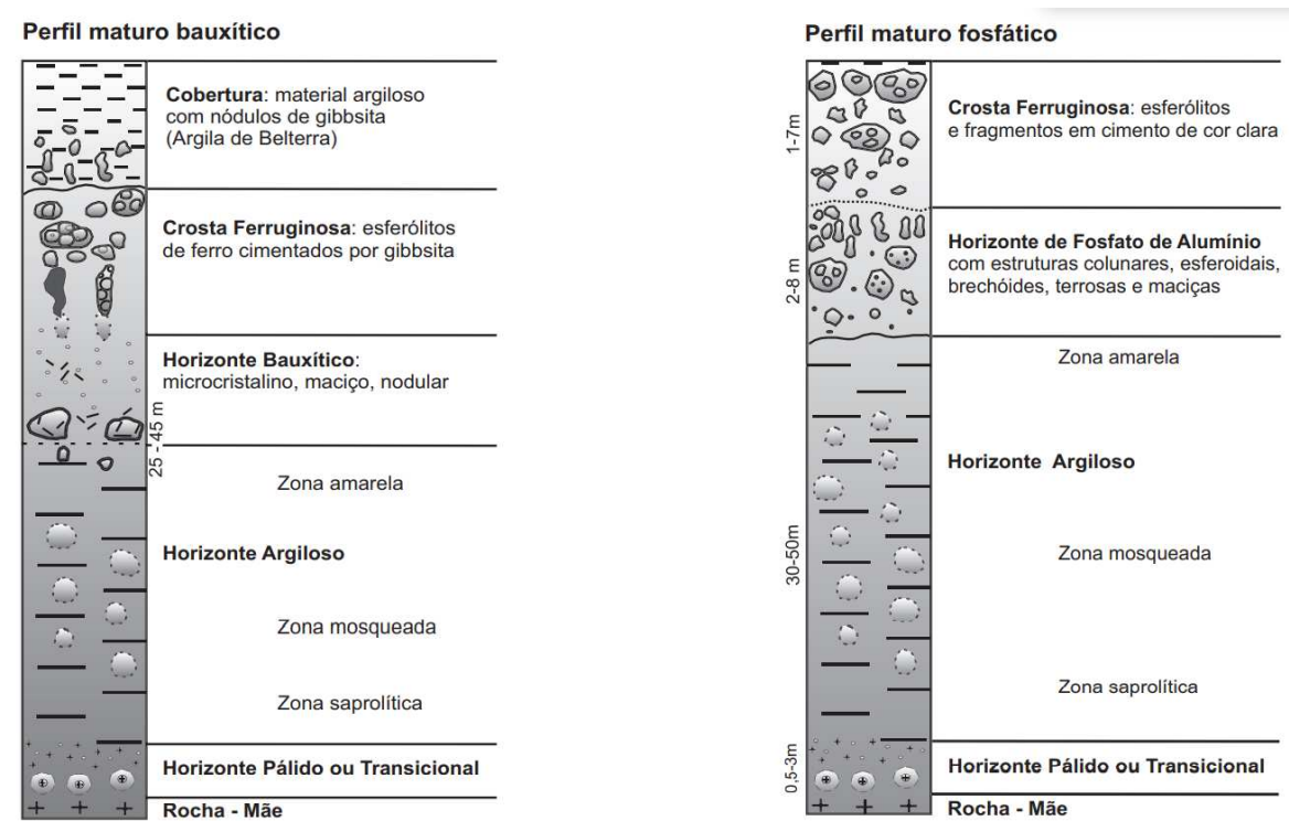
Figura 16 – Perfis geológicos simplificados de lateritas maduras autóctones na Amazônia.
