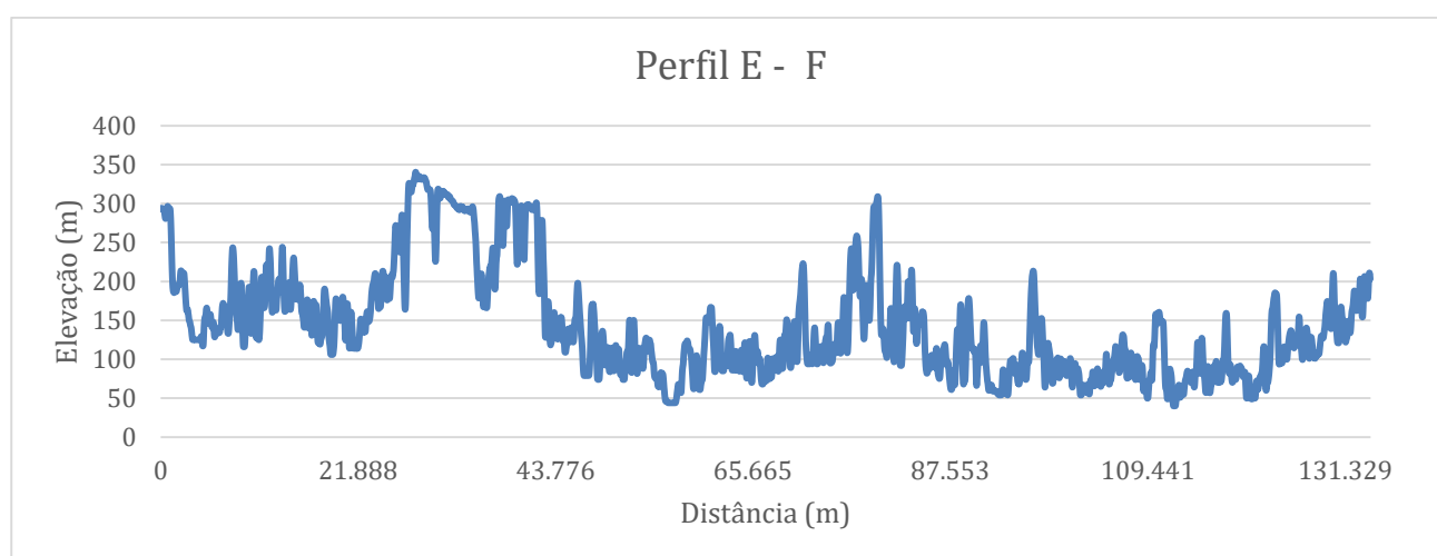
Figura 51 – Perfil topográfico E-F.
