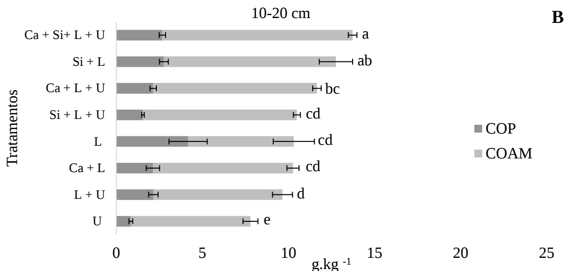
Figura 4 - Frações do carbono; carbono orgânico particulado (COP) e carbono orgânico associado aos minerais (COAM) nas profundidades de A) 0 – 10 cm e B) 10 - 20 cm (g.kg -1 ). O carbono orgânico total (COT) é representado pela soma das duas frações. Tratamentos 1) U (ureia); 2) L (leguminosas); 3) L + U (leguminosas + ureia); 4) Ca + L (cálcio + leguminosas); 5) Si + L (silício + leguminosas); 6) Ca + L + U (cálcio + leguminosas + ureia); 7) Si + L + U (silício + leguminosas + ureia) e; 8) Ca + Si + L + U (cálcio + silício + leguminosas + ureia). Médias seguidas por letras diferentes indicam diferenças entre si pelo teste de Tukey a 5% de probabilidade.
