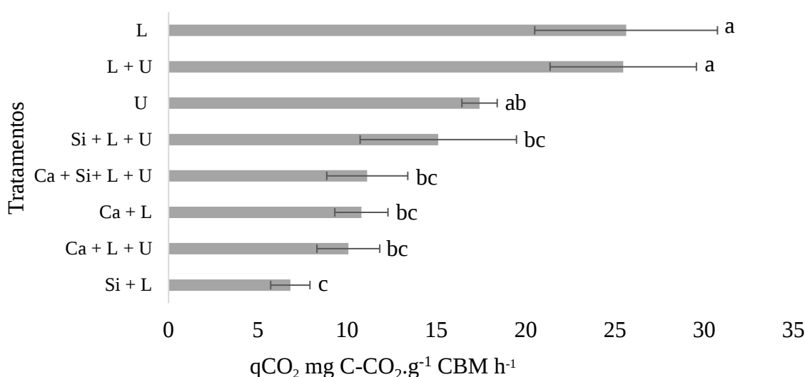
Figura 2 - Quociente metabólico ( mg\ C-CO_2.g^{-1}\ CBM\ h^{-1} ) na profundidade de 0-10 cm. Tratamentos 1) U (ureia); 2) L (leguminosas); 3) L + U (leguminosas + ureia); 4) Ca + L (cálcio + leguminosas); 5) Si + L (silício + leguminosas); 6) Ca + L + U (cálcio + leguminosas + ureia); 7) Si + L + U (silício + leguminosas + ureia) e; 8) Ca + Si + L + U (cálcio + silício + leguminosas + ureia). Médias seguidas por letras diferentes indicam diferenças entre si pelo teste de Tukey a 5% de probabilidade.
