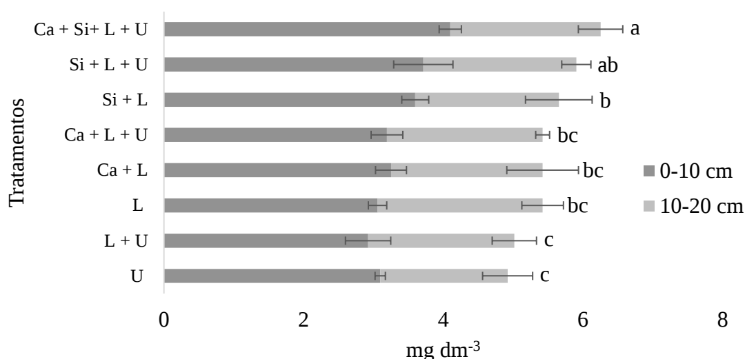
Figura 6. Teores de silício disponível ( \text{mg dm}^{-3} ) no solo nas profundidades de 0-10 cm e 10-20 cm. Tratamentos 1) U (ureia); 2) L (leguminosas); 3) L + U (leguminosas + ureia); 4) Ca + L (cálcio + leguminosas); 5) Si + L (silício + leguminosas); 6) Ca + L + U (cálcio + leguminosas + ureia); 7) Si + L + U (silício + leguminosas + ureia) e; 8) Ca + Si + L + U (cálcio + silício + leguminosas + ureia). Médias seguidas por letras diferentes indicam diferenças entre si pelo teste de LSD a 5% de probabilidade.
