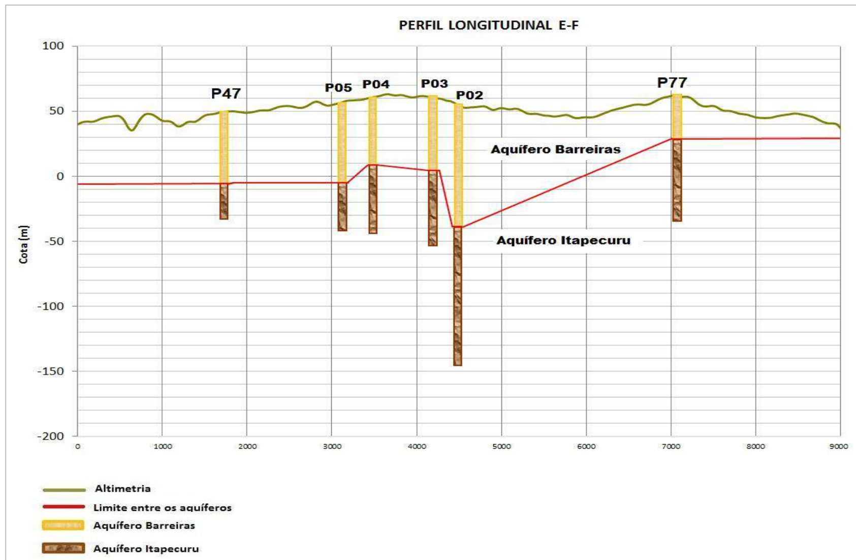
Figura 47 - Perfil litológico do traçado E-F dos poços tubulares localizados na bacia do rio Tibiri e adjacências, em São Luís – MA.
