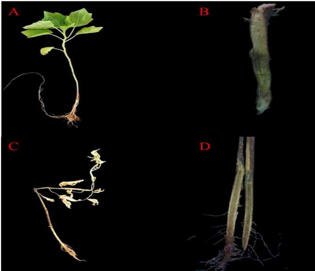
Figura 20- A – Planta de Jurubeba peito de moça com aspecto saudável; B – Caule da jurubeba peito-de-moça sem escurecimento vascular; C- Planta de tomate com murcha bacteriana; D – Caule do tomateiro com escurecimento vascular.
