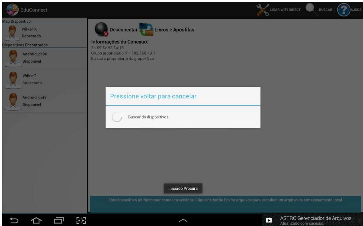
Figura 4.18 - Interação Usuário-sistema
