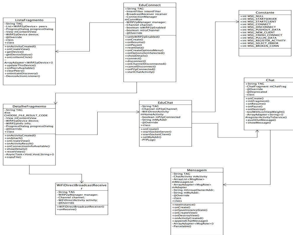
Figura 4.9 - Diagrama de Classe Módulo Chat
