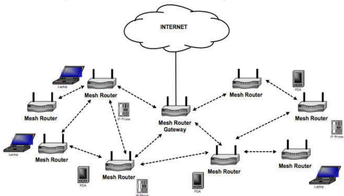
Figura 3.1 - Redes mesh
