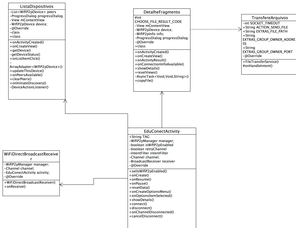
Figura 4.5 – Diagrama de Classe módulo Arquivos
