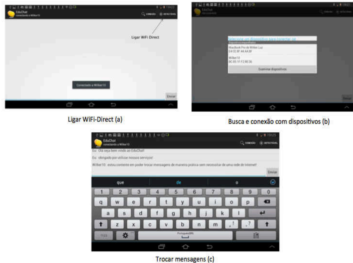
Figura 4.8 - Módulo EduChat
