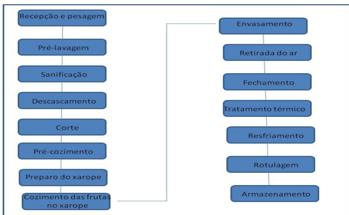
Figura (05) – Fluxograma da produção de doces da Coopral.
