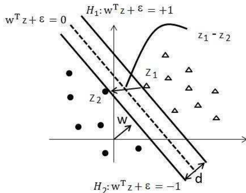
Figura 8 - Hiperplano ótimo, com dois vetores de suporte H_1 e H_2
