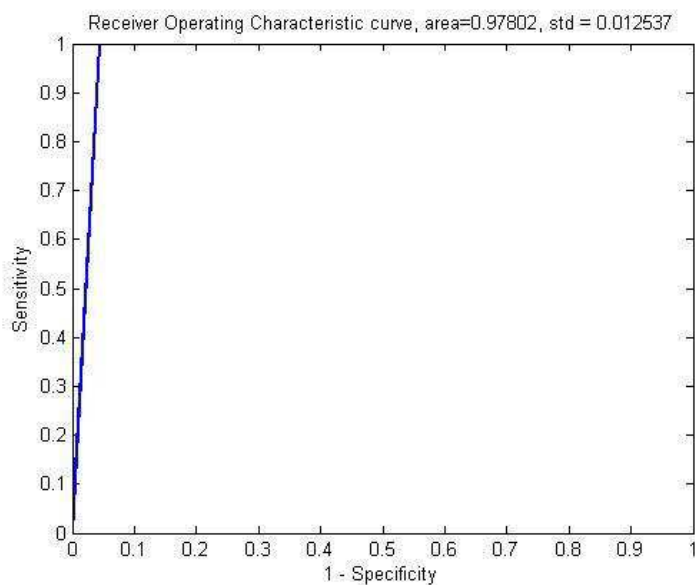
Figura 11 – Área sob a curva ROC para o vetor de 10 características
