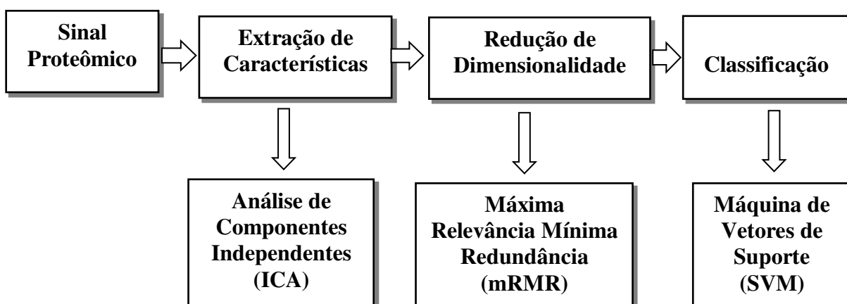
Figura 9 - Diagrama em blocos do método proposto
