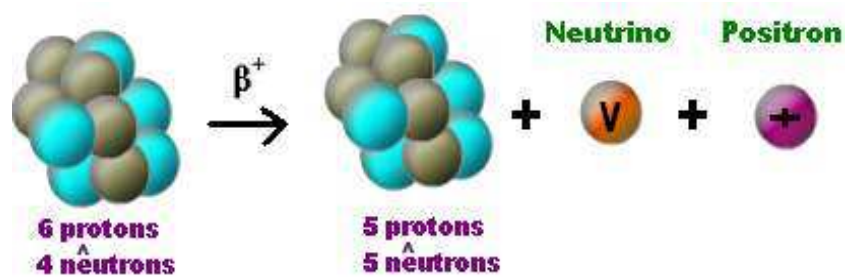
Figura 9- Decaimento beta mais
