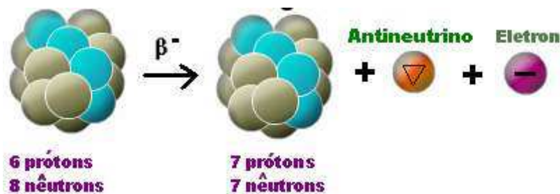
Figura 8- Decaimento beta menos
