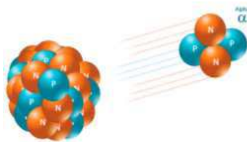
Figura 7- Decaimento Alfa
