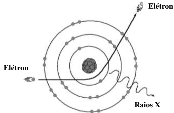
Figura 13- Produção de raios X por bremstrahlung
