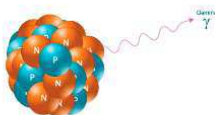
Figura 10- Emissão gama
