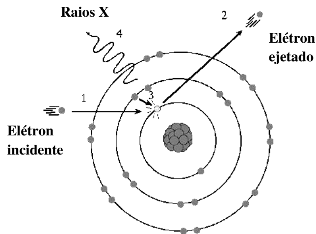
Figura 14- Espectro característico de raios X
