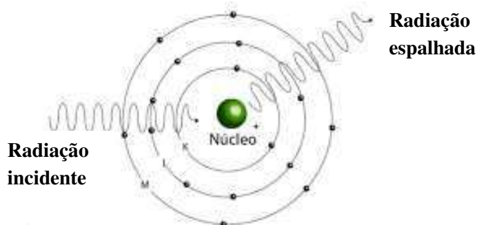
Figura 3- Espalhamento Rayleigh
