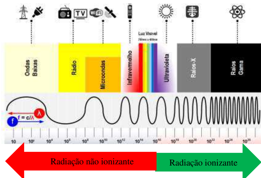
Figura 11- Espectro eletromagnético
