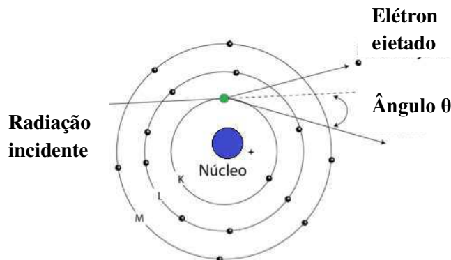
Figura 4- Espalhamento Compton
