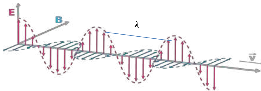
Figura 1- Representação vetorial de uma onda eletromagnética
