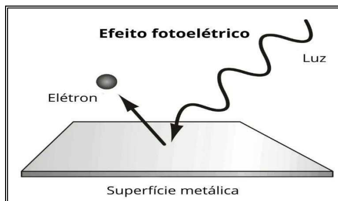
FIGURA 2-EFEITO FOTOELÉTRICO
