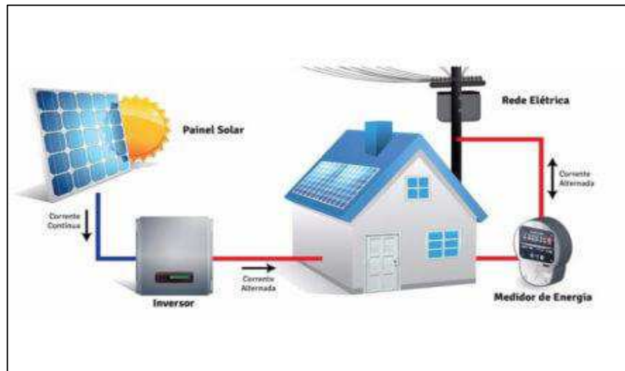
FIGURA 11: SISTEMA ON-GRID
