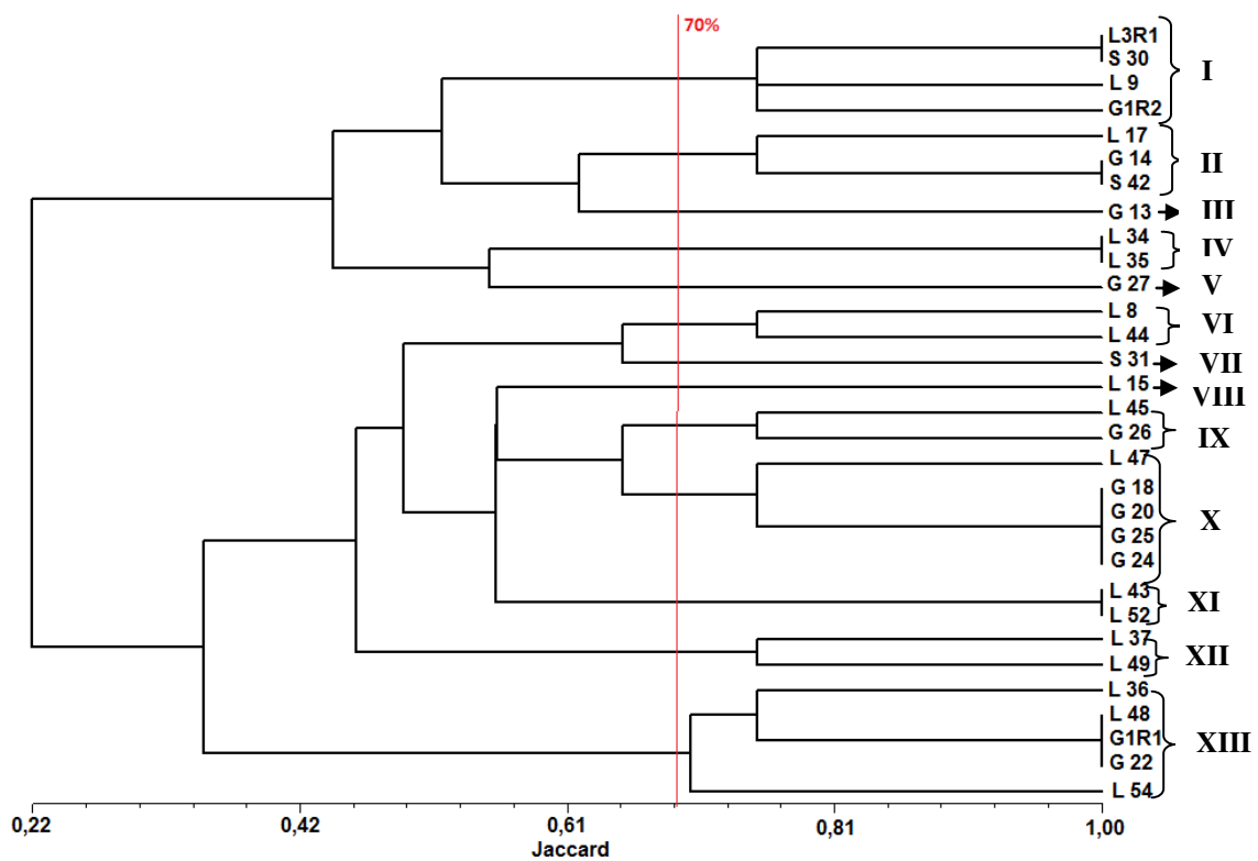
Figura 1. Dendrograma de similaridade com base em características fenotípicas dos isolados de bactérias que nodulam leucena, gliricidia e sombreiro, oriundos de solo proveniente do Centro-Norte Maranhense. * L = isolados provenientes de leucena, S = isolados provenientes de sombreiro e G = isolados provenientes de gliricidia.
