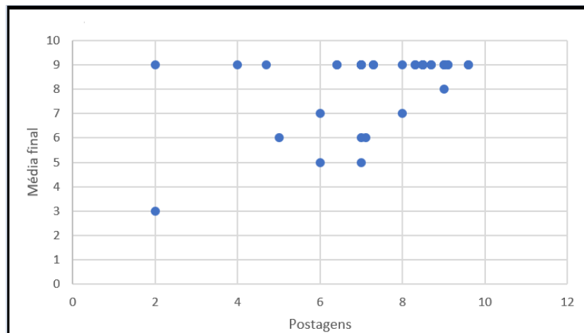
Figura 6 - gráfico de dispersão da quantidade de postagens
